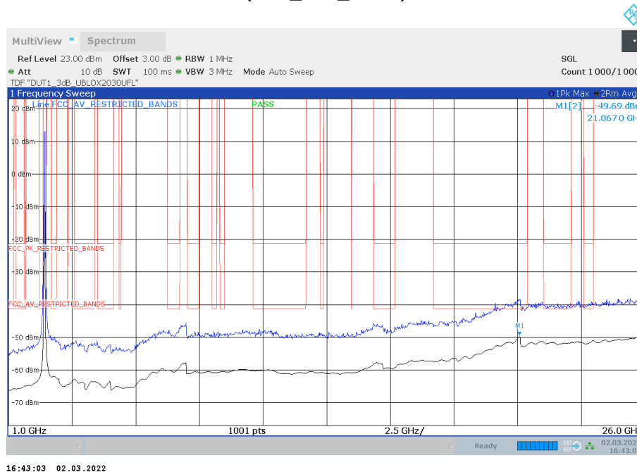
Antenna A
