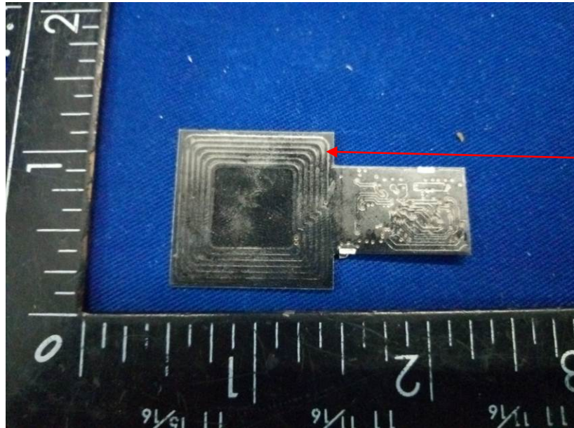
RFID Antenna
