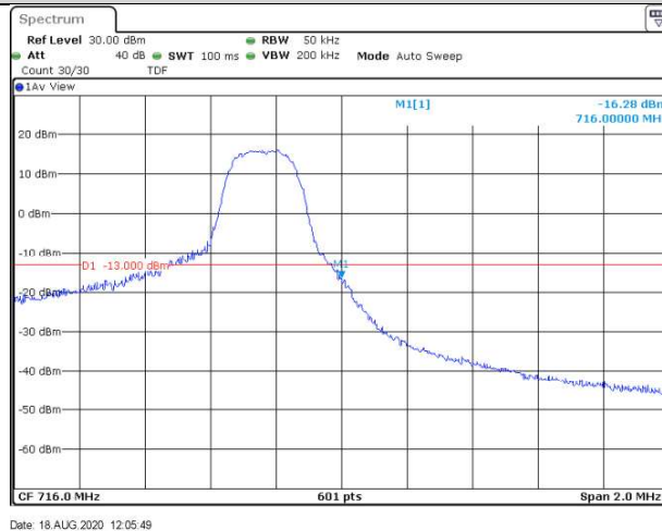
Band12-3MHz-QPSK-23165-15RB#0
