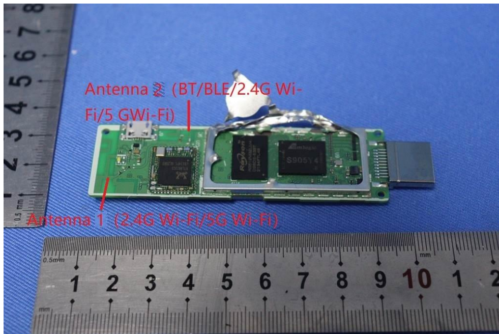
Antenna
