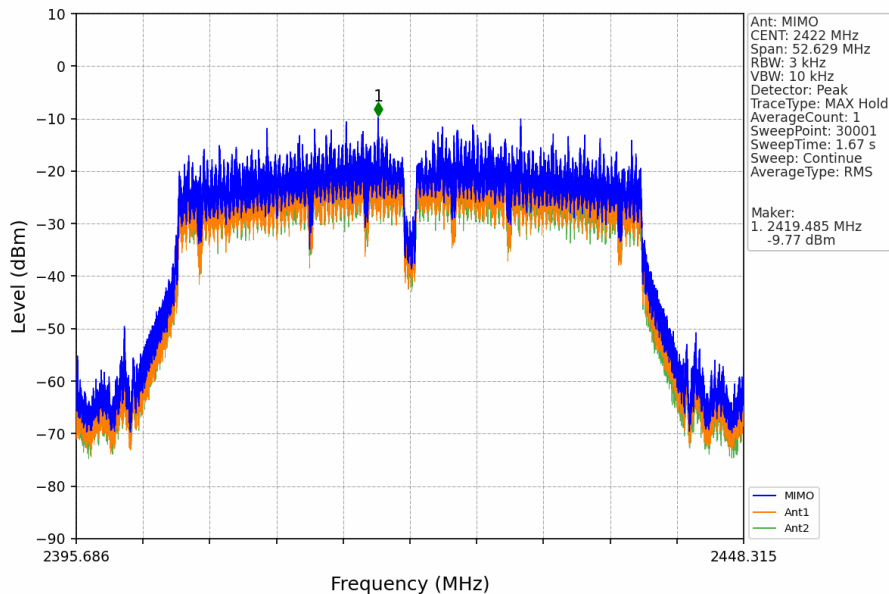
802.11n(HT40)_LCH_2422MHz_MIMO_NTNV
