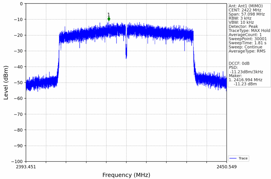
802.11ax(HEW40)_LCH_2422MHz_RU484_Left_Ant1 (MIMO)_NTNV
