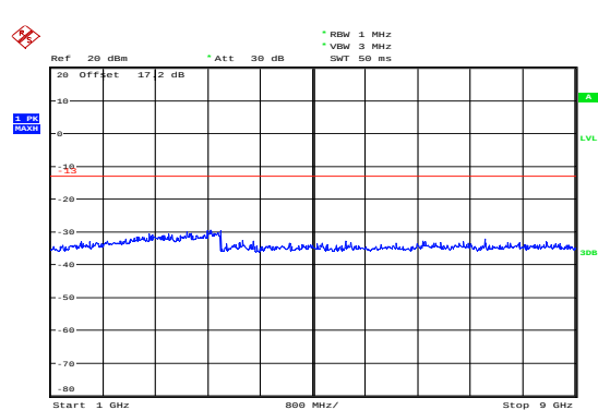
GSM 850 CH-Low 1GHz ~ 9GHz
