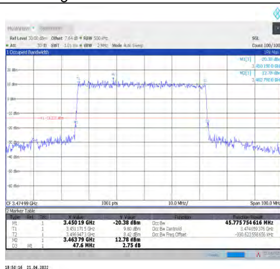
1-N78-3450-3550--30-50-L-3-DFT-16QAM-Out_Fu ll-128@0-Ant1-45.776-47.600-≤50-PASS
