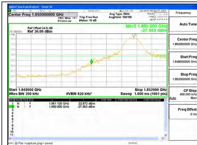
Band2 / 20MHz / Low CH / QPSK / 1 RB
