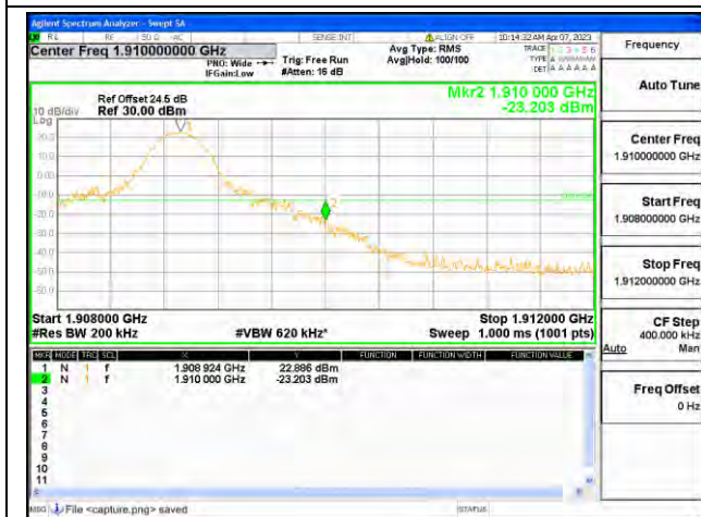
Band2 / 20MHz / High CH / QPSK / 1 RB
