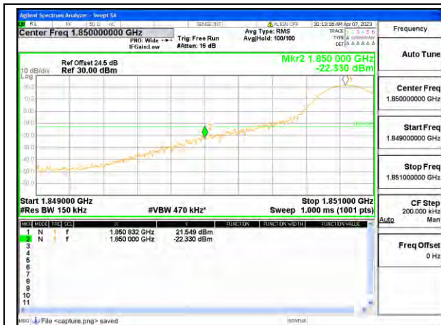
Band2 / 15MHz / Low CH / QPSK / 1 RB
