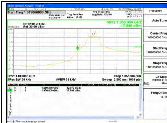
Band2 / 3MHz / Low CH / QPSK / 1 RB
