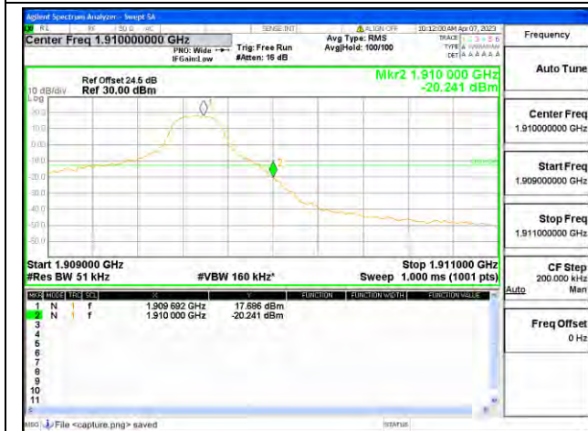
Band2 / 5MHz / High CH / QPSK / 1 RB
