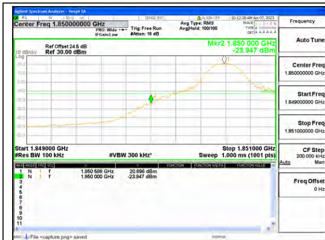
Band2 / 10MHz / Low CH / QPSK / 1 RB
