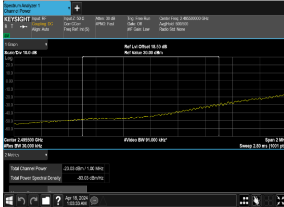
N41(100M)_DFT-s-OFDM_QPSK_ Edge_1RB_Left_Low_CH_CHP_PASS
