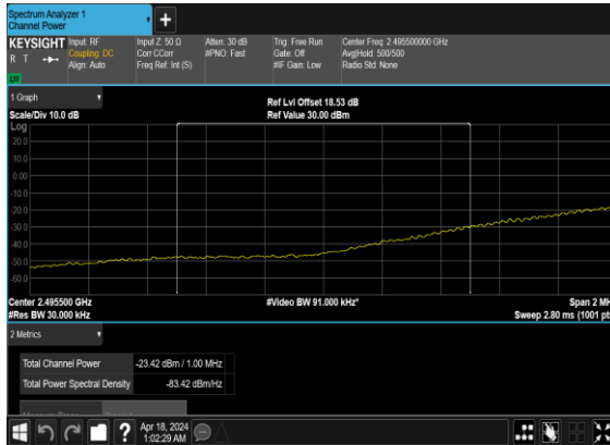
N41(100M)_DFT-s-OFDM_BPSK_ Edge_1RB_Left_Low_CH_CHP_PASS
