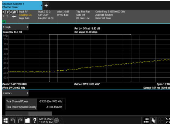
N41(60M)_DFT-s-OFDM_BPSK_ Edge_1RB_Left_Low_CH_CHP_PASS
