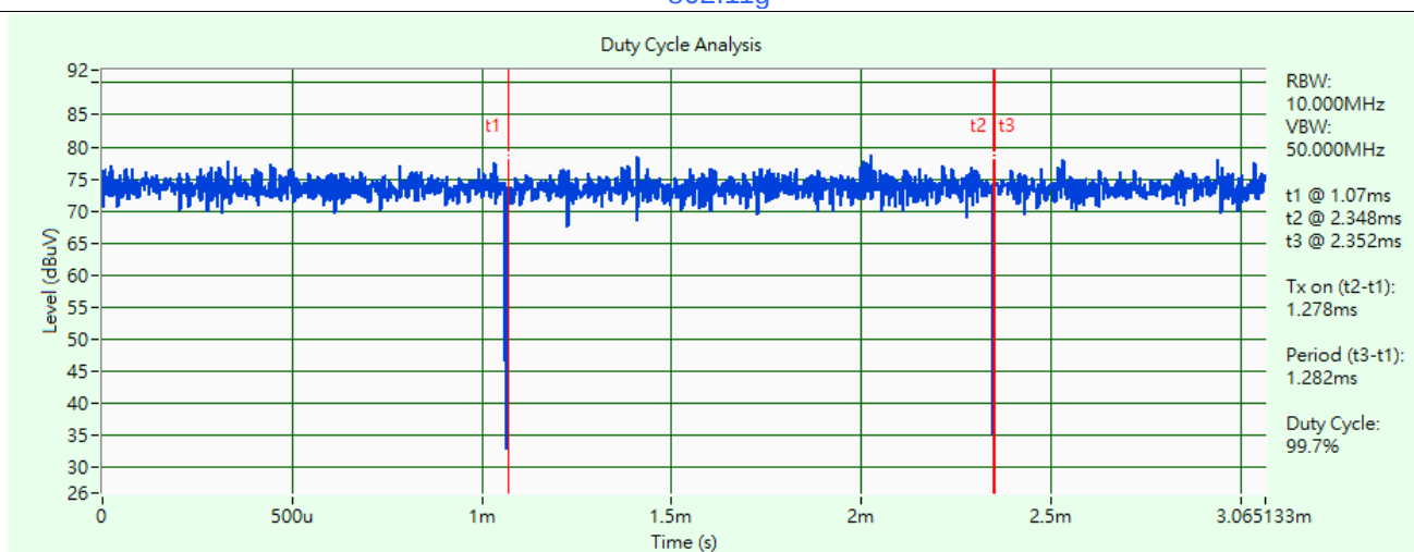
802.11n (HT20)
