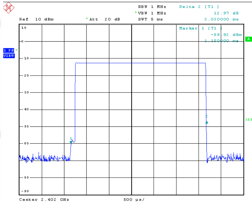
2402 MHz_DH5
