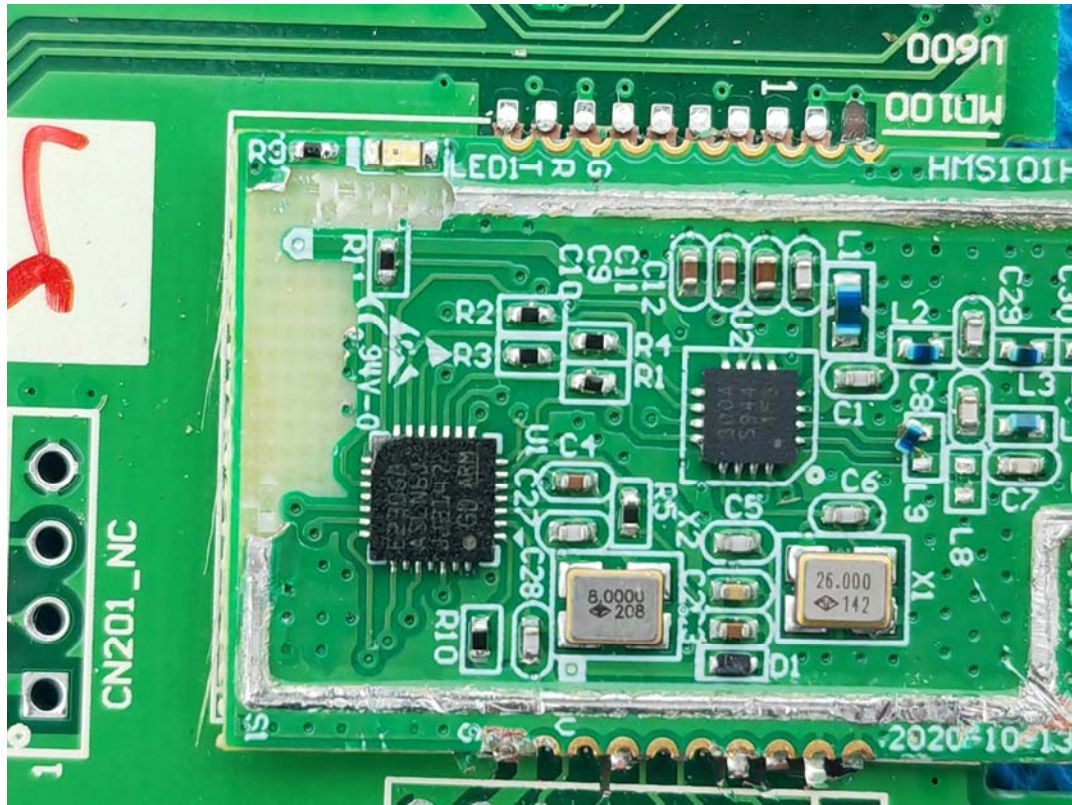
FHSS chip
