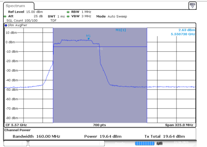
MIMO B-802.11ax/be160-Ch114-5570MHz-MCS0
