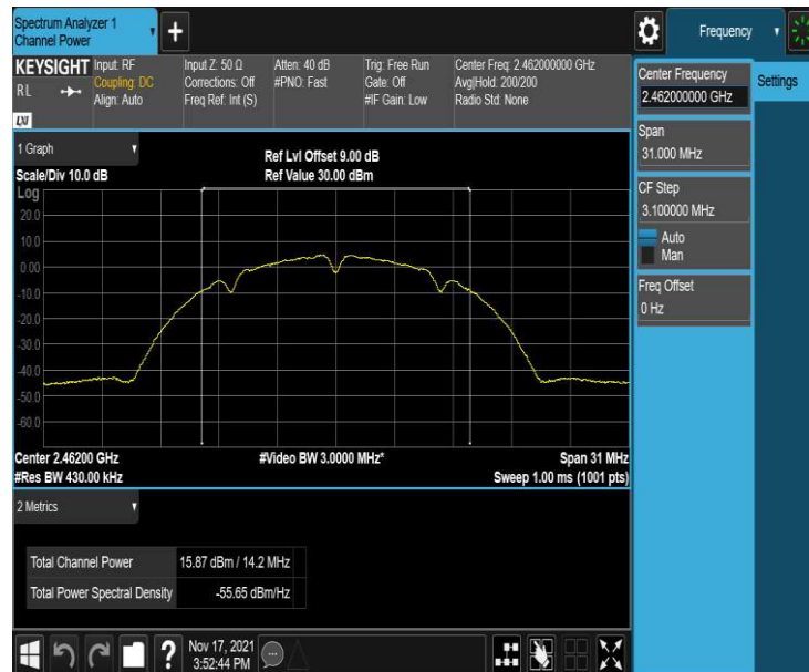
11B_Ant1_2462
