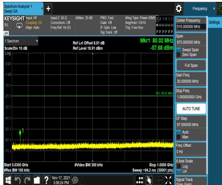
11G_Ant1_2412_30~1000
