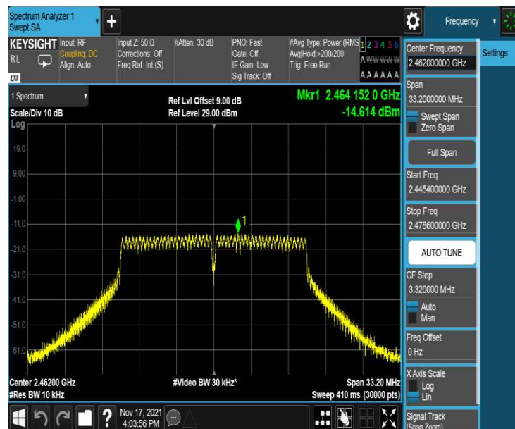
11G_Ant1_2462
