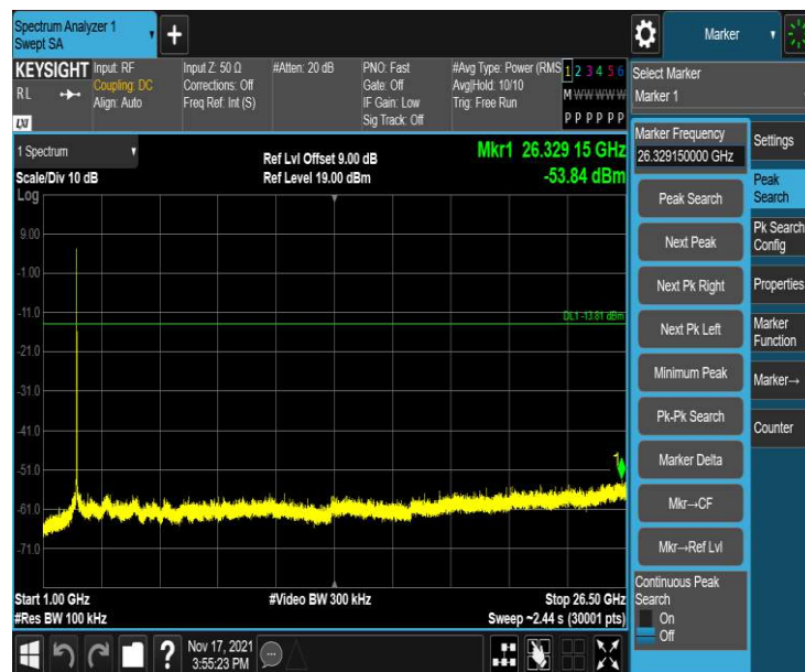
11B_Ant1_2462_1000~26500
