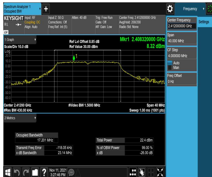
11G_Ant1_2412
