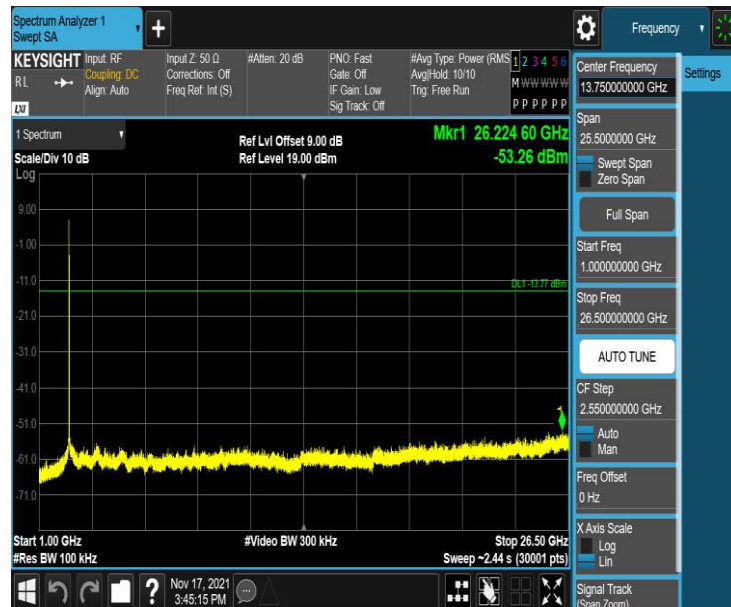
11B_Ant1_2437_1000~26500
