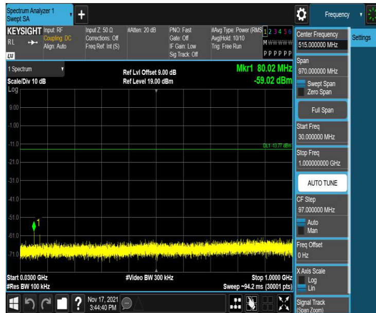
11B_Ant1_2437_30~1000
