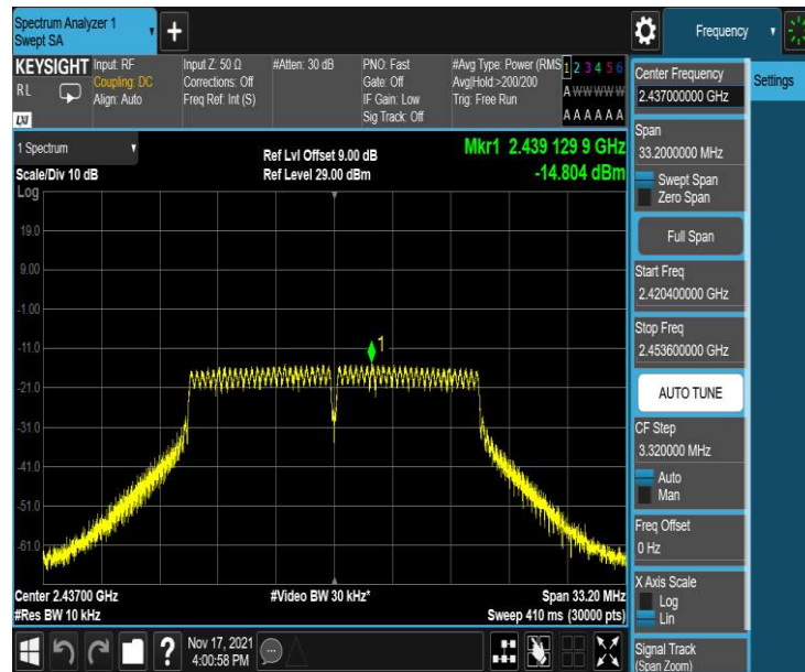
11G_Ant1_2437
