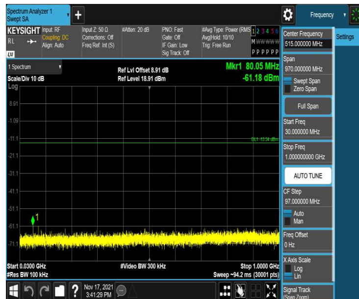
11B_Ant1_2412_30~1000
