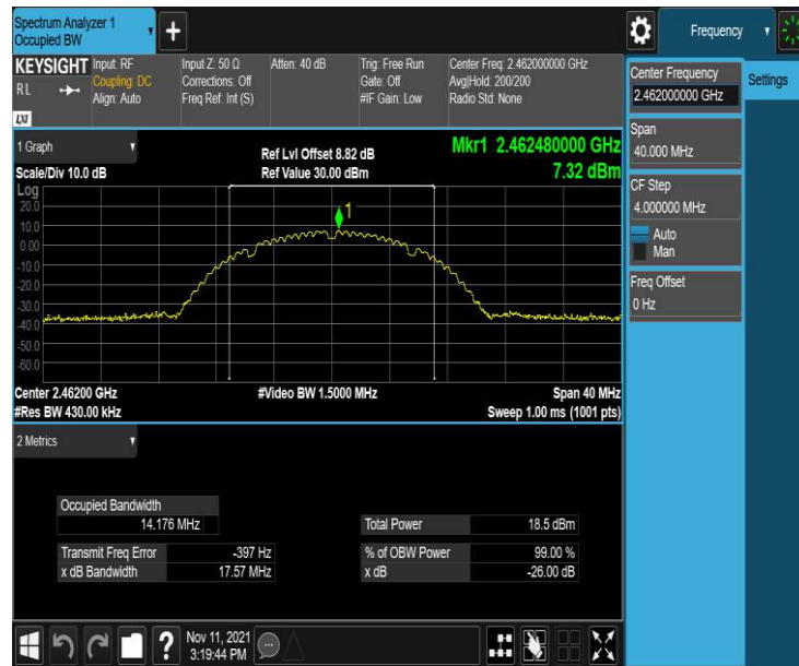
11B_Ant1_2462
