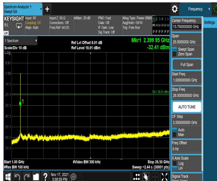
11G_Ant1_2412_1000~26500
