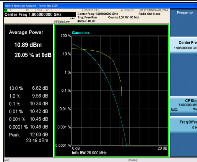
Band25-20MHz-16QAM-26590-1-0-Low-10.34-&lt;=13-PASS
