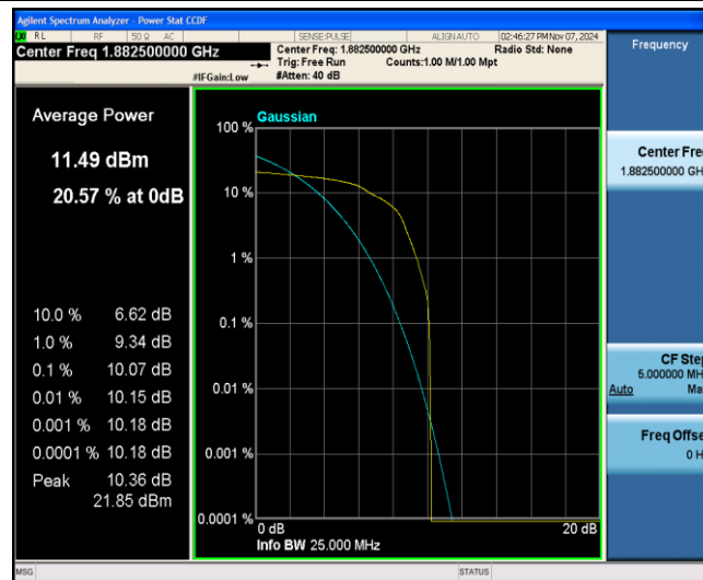
Band25-20MHz-16QAM-26365-1-0-Low-10.07-&lt;=13-PASS
