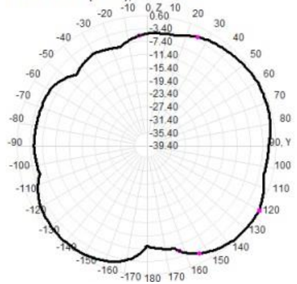
2500.0MHz Total(E2-YZ), Max= 0.51dBi
