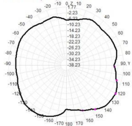
2400.0MHz Total(E2-YZ), Max= 1.26dBi
