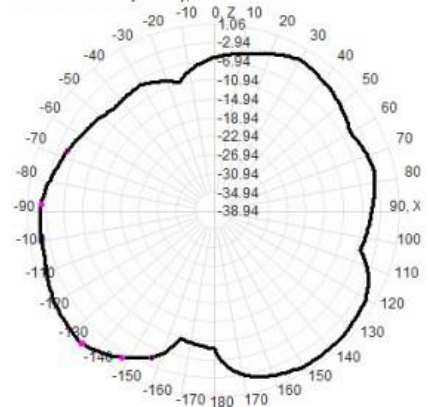
2450.0MHz Total(E1-XZ), Max= 1.06dBi
