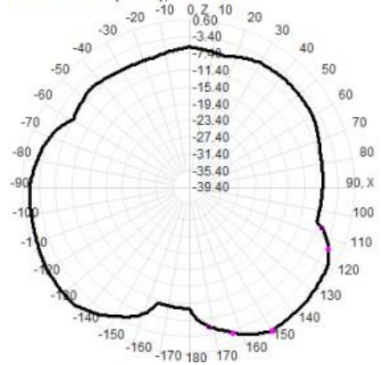
2500.0MHz Total(E1-XZ), Max= 0.24dBi
