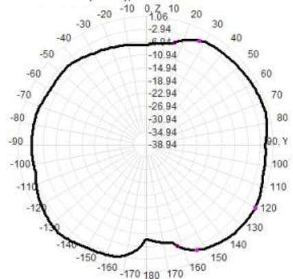
2450.0MHz Total(E2-YZ), Max= 0.58dBi
