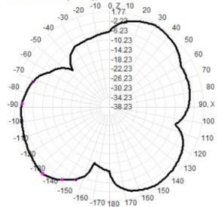
2400.0MHz Total(E1-XZ), Max= 1.55dBi
