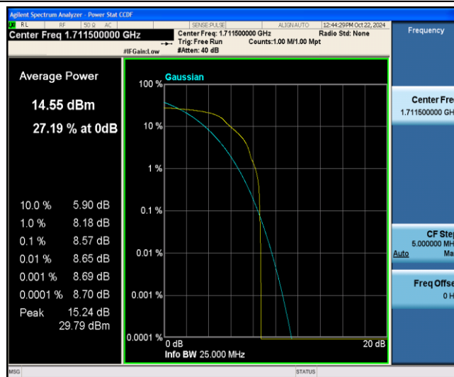
Band4-3MHz-QPSK-19965-1-0-Low-8.57-&lt;=13-PASS
