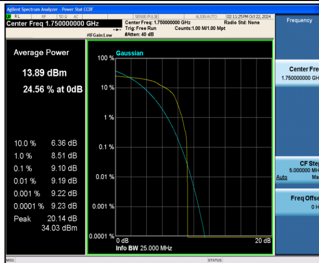
Band4-10MHz-16QAM-20350-1-0-Low-9.10-=&lt;=13-PASS
