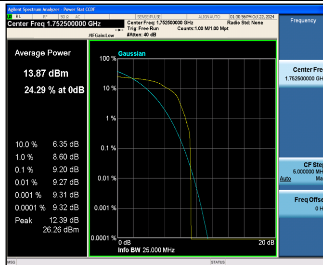
Band4-5MHz-16QAM-20375-1-0-Low-9.20-&lt;=13-PASS
