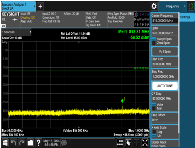
BLE_2M-Ant1-2440-30~1000-PASS
