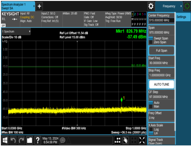
BLE_2M-Ant1-2480-30~1000-PASS
