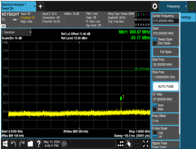
BLE_2M-Ant1-2402-30~1000-PASS
