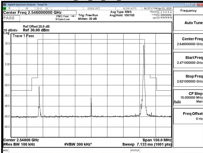
Mask_n41_CH_Low_1RBmax
