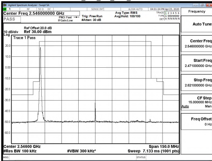
Mask_n41_CH_Low_1RBmax
