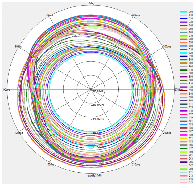
900RX/PCS1900/WCDMA B2/LTE B2 Theta=90deg
