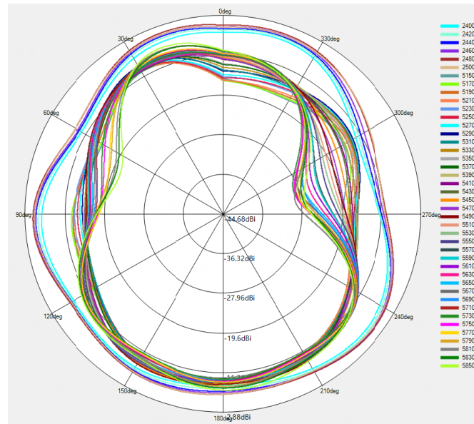
BT/WIFI-2.4G & 5G \Phi=90^\circ
