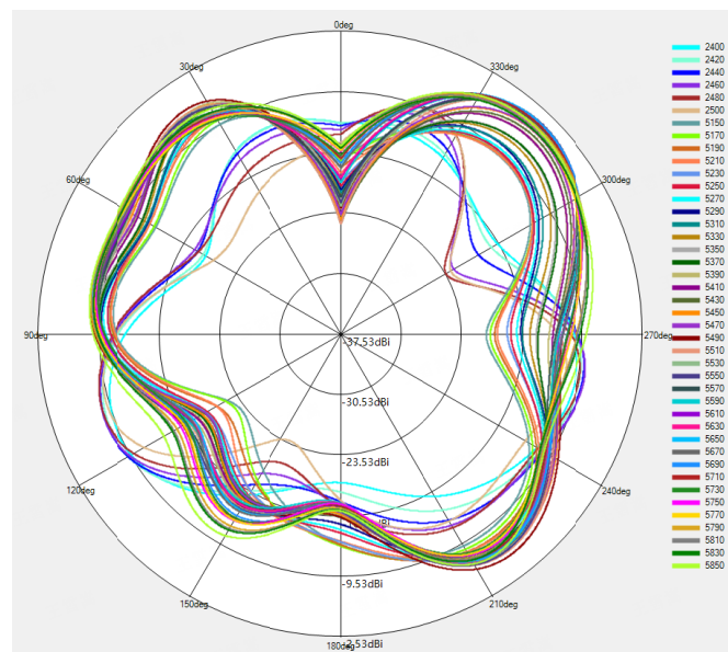
BT/WIFI-2.4G & 5G \Theta=90^\circ
