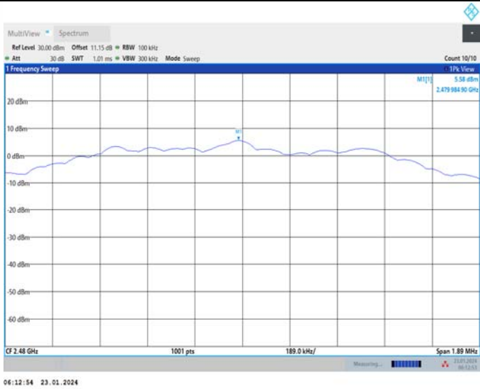
BLE_2M_Ant1_2480
