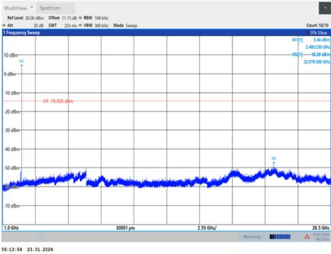
BLE_2M_Ant1_2480_1000~26500
