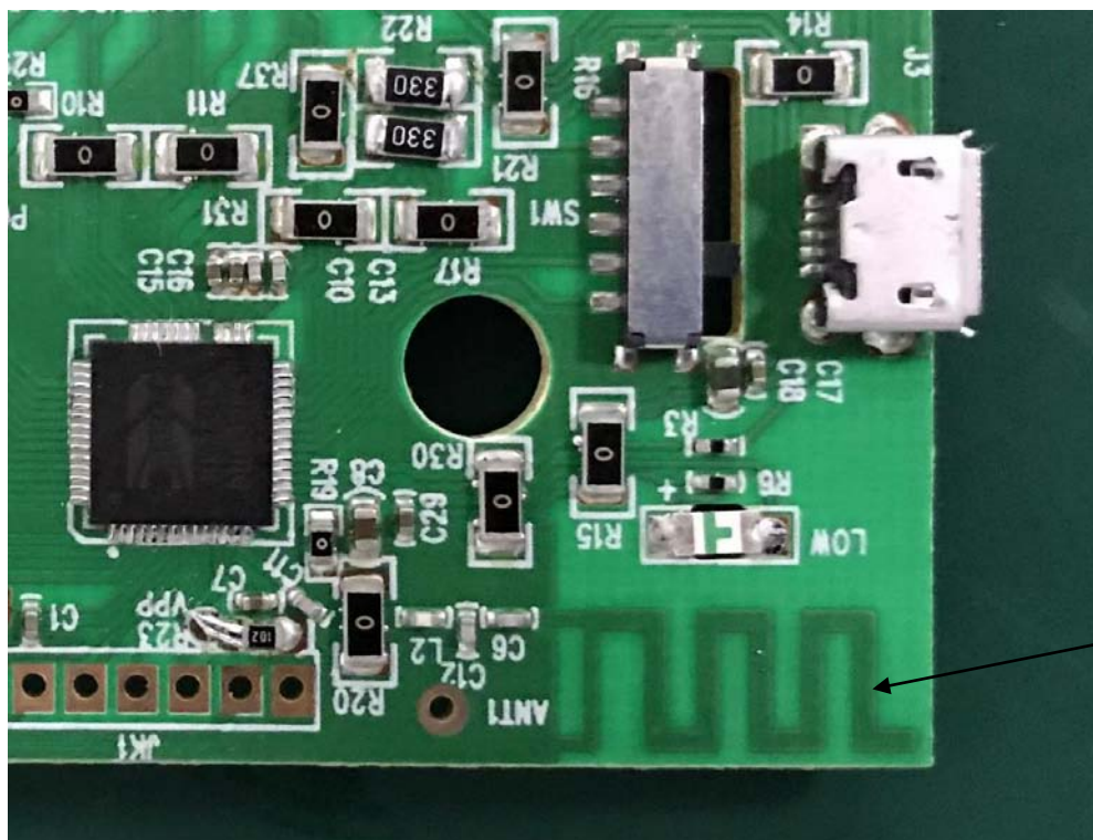
Antenna
