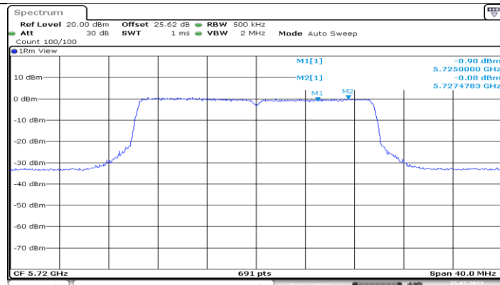
11BE20MIMO_Ant4_5720_UNII-3
