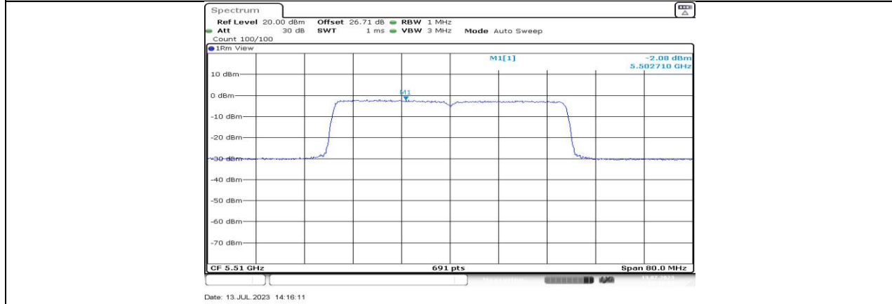
11BE40MIMO_Ant1_5510
