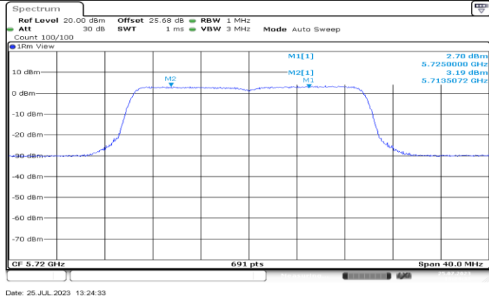
11BE20MIMO_Ant3_5720_UNII-2C
