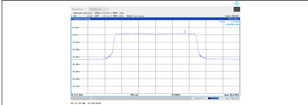
11BE40MIMO_Ant4_5310
