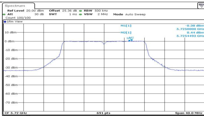
11A-CDD_Ant3_5720_UNII-3
