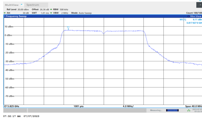
11A-CDD_Ant2_5825
