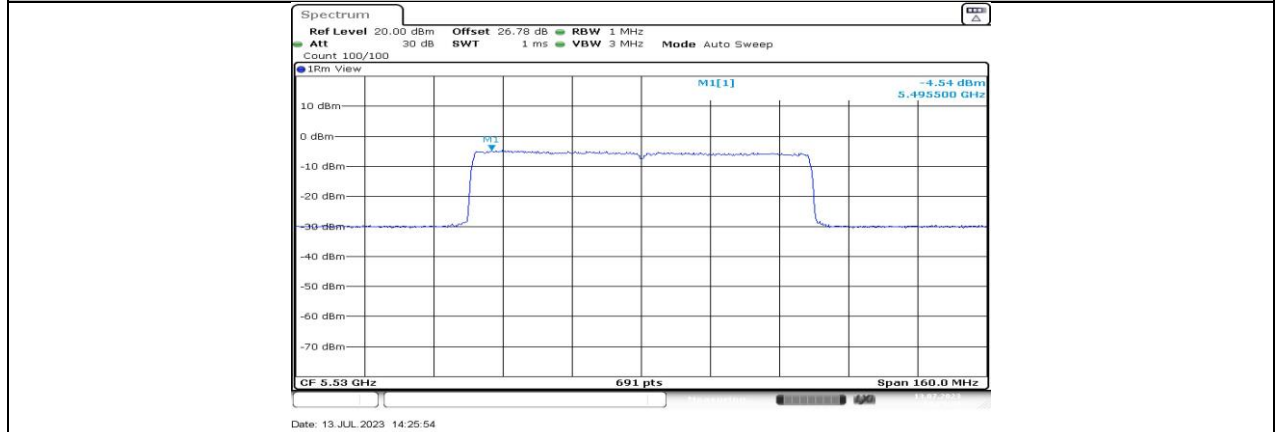
11BE80MIMO_Ant1_5530
