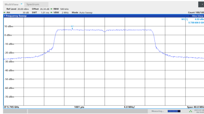
11BE20MIMO_Ant1_5745
