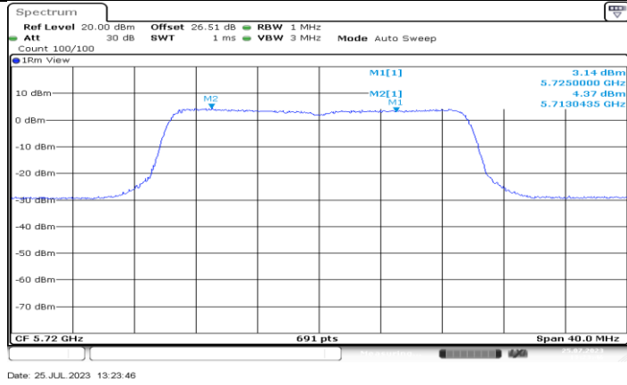
11BE20MIMO_Ant2_5720_UNII-2C
