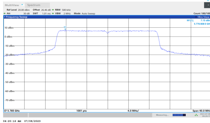
11BE20MIMO_Ant1_5785
