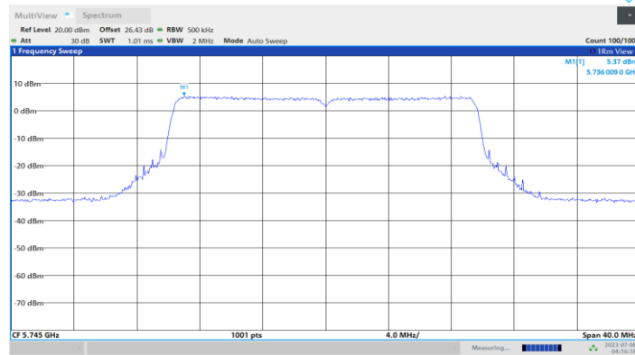
11BE20MIMO_Ant2_5745
