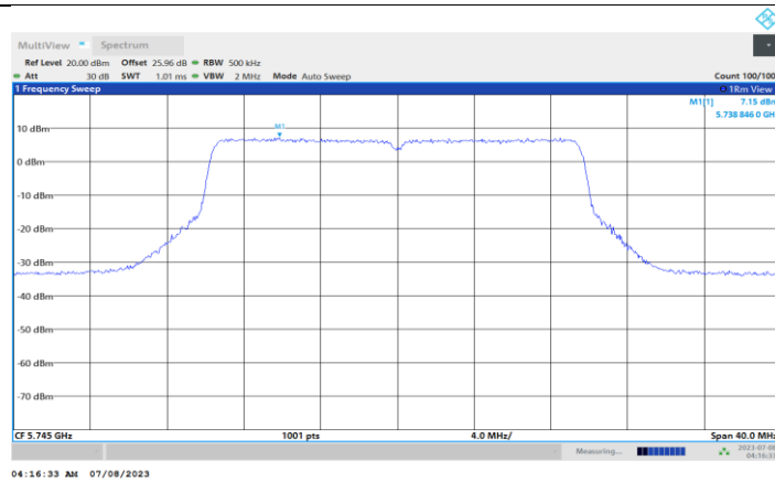
11BE20MIMO_Ant3_5745
