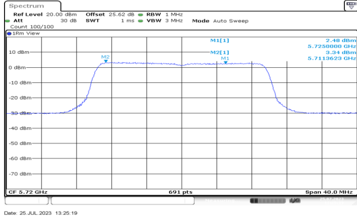
11BE20MIMO_Ant4_5720_UNII-2C
