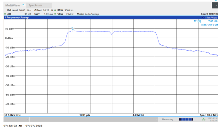
11A-CDD_Ant1_5825
