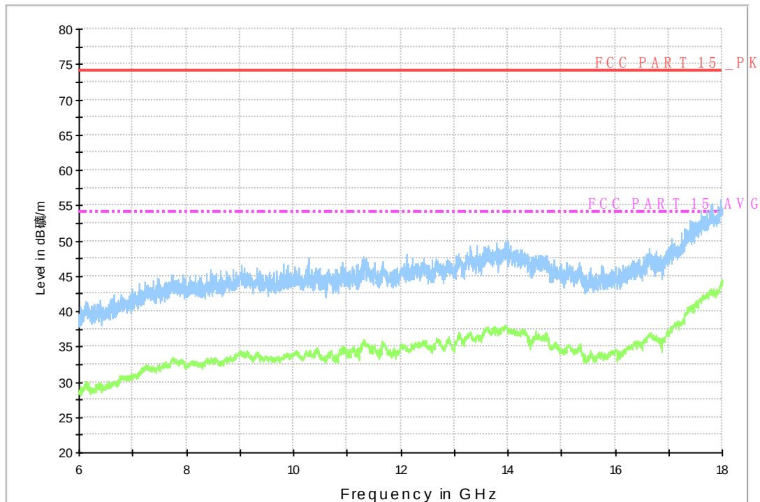
Normal RE_6G-18GHz
