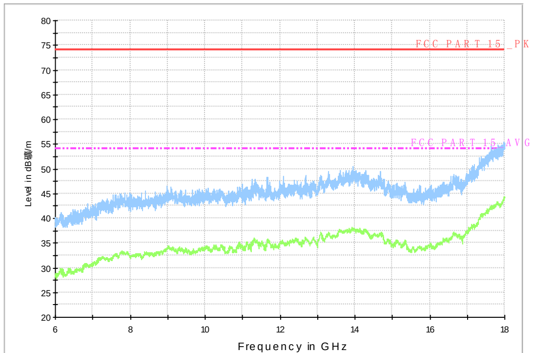
Normal RE_6G-18GHz
