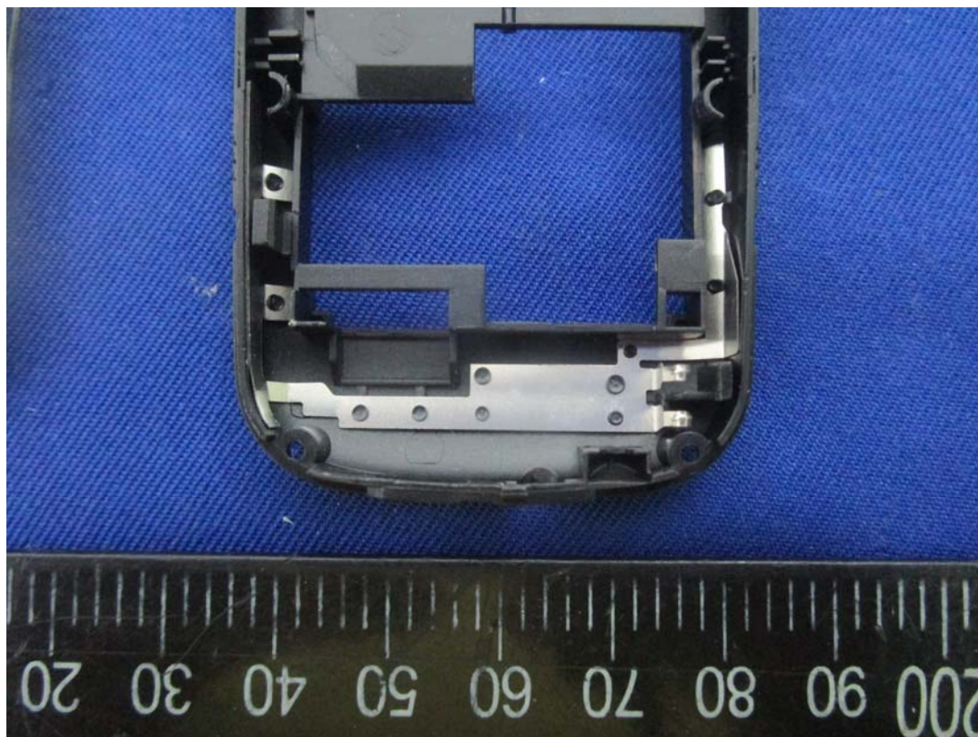
GSM Antenna
