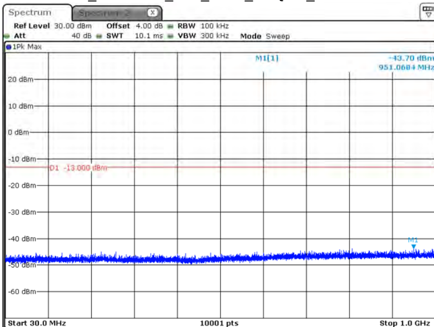
B66_CH132072_20M_1RB0_16-QAM_Below 1G
