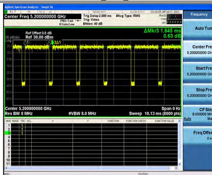
802.11a_Ant2_5200
