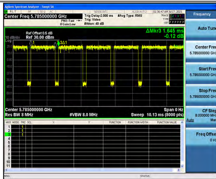
802.11a_Ant2_5785
