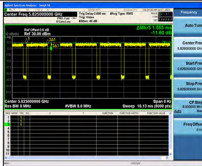
802.11n(HT20)_Ant2_5825
