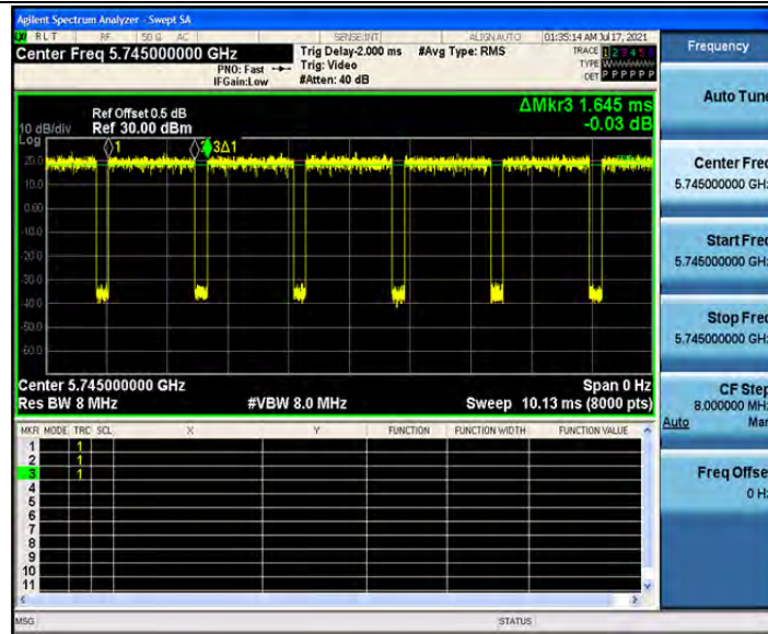
802.11a_Ant2_5745
