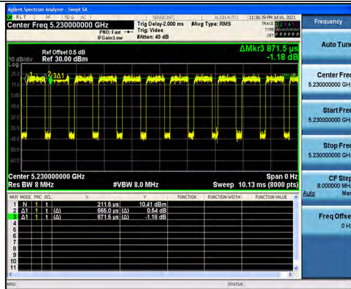
802.11n(HT40)_Ant2_5230
