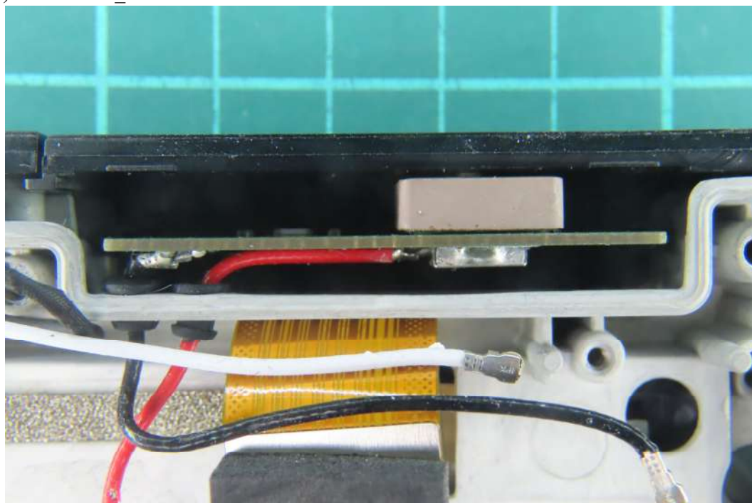
(46) EUT Photo_WLAN AUX Antenna
