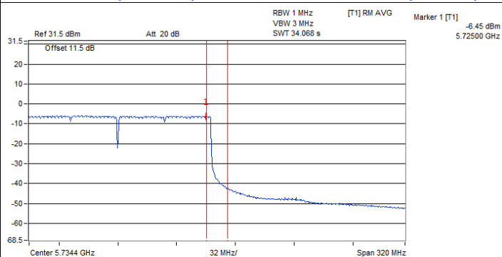
802.11be (EHT240) / Chain 0 : CH 114+138 (U-NII-3)
