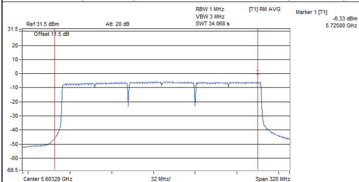
802.11be (EHT240) / Chain 0 : CH 114+138 (U-NII-2C)
