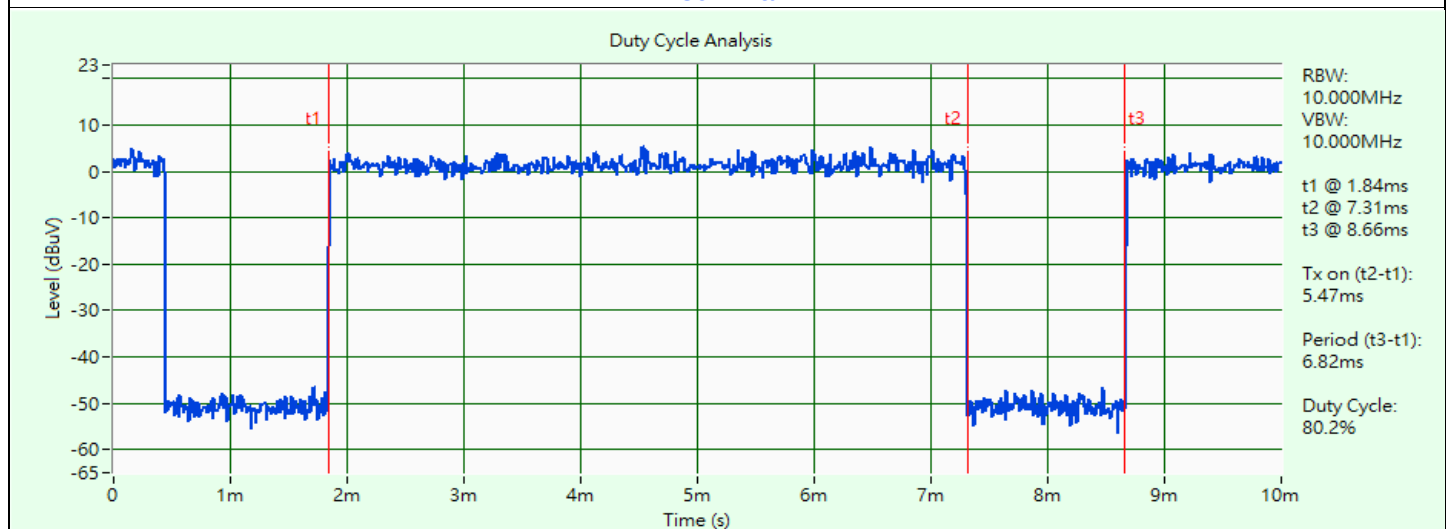
802.11be (EHT20)
