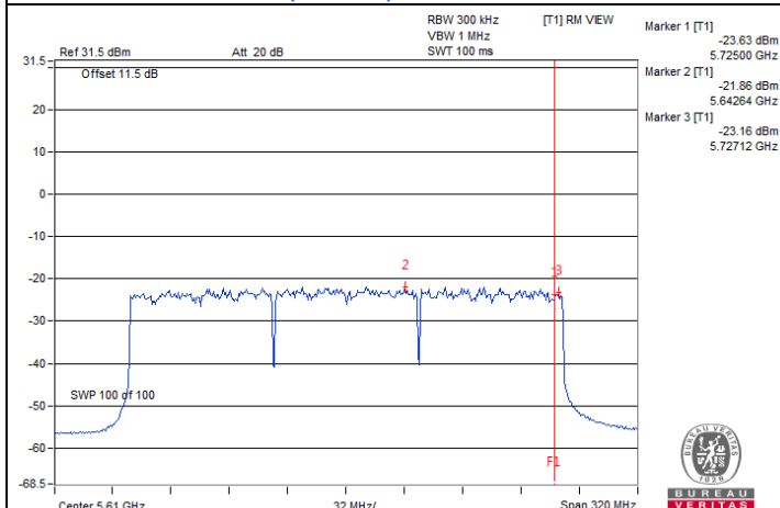
802.11be (EHT240) / Chain 0 : CH 114+138
