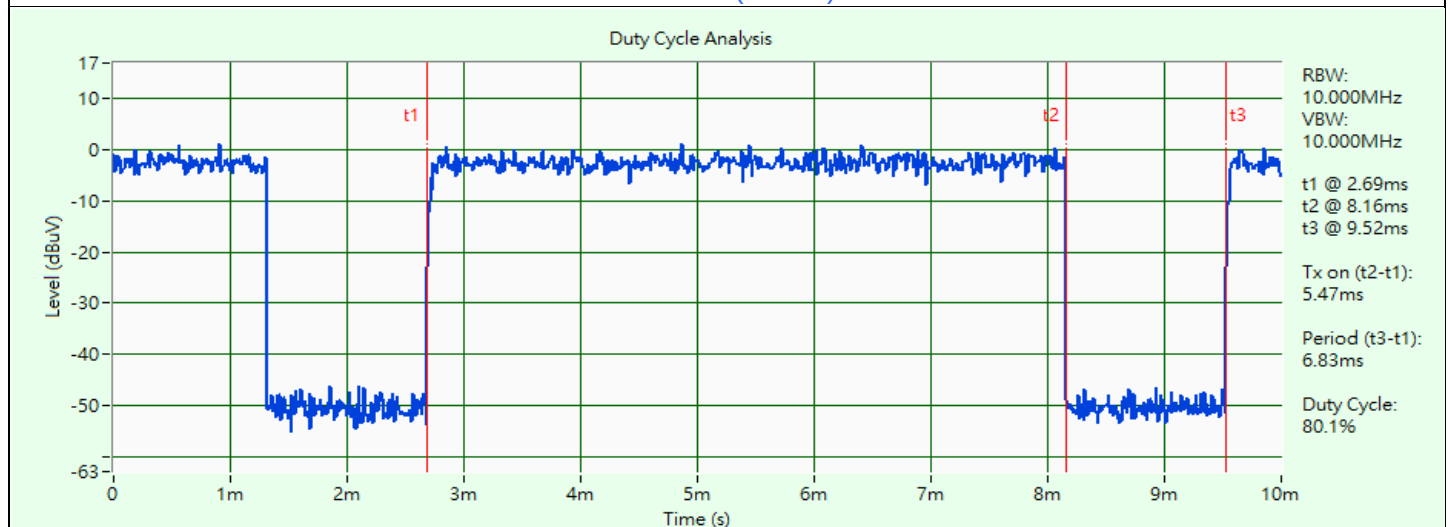
802.11be (EHT40)
