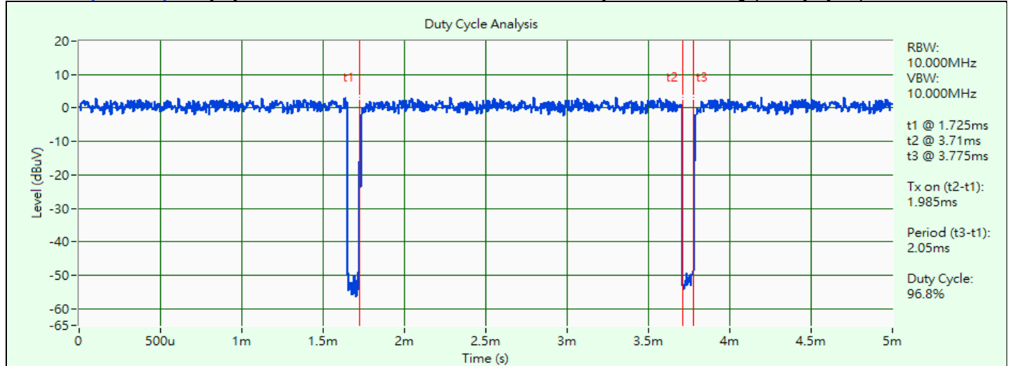
802.11a
