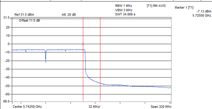
802.11be (EHT240) / Chain 1 : CH 114+138 (U-NII-3)
