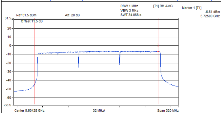
802.11be (EHT240) / Chain 1 : CH 114+138 (U-NII-2C)
