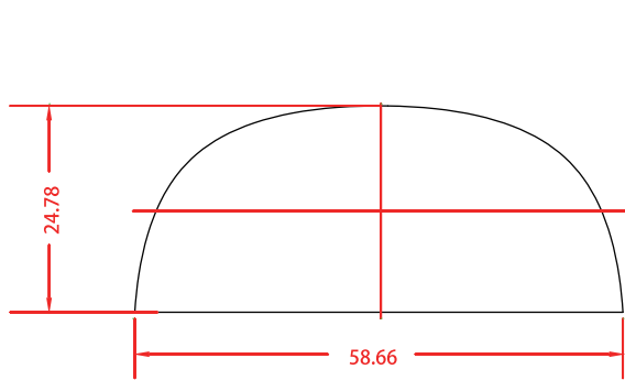
结构尺寸图
