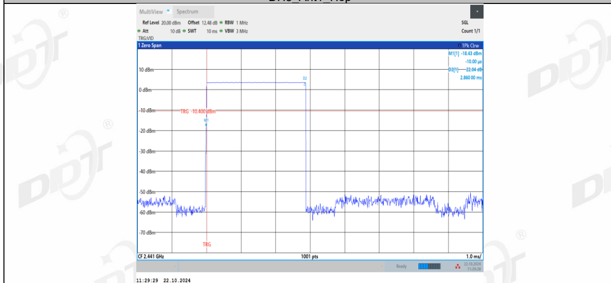
DH5_Ant1_Hop
