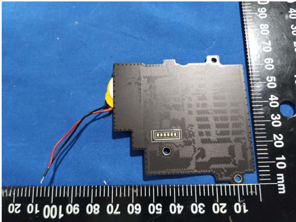
4G Antenna
