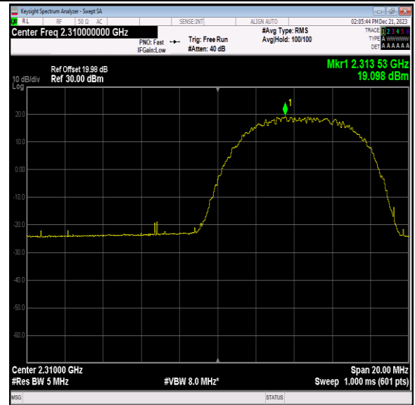
40(2305-2315)-10MHz-64QAM-38750-1RB#49-PASS
