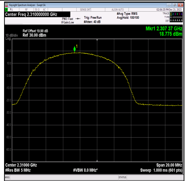
40(2305-2315)-10MHz-64QAM-38750-25RB#12-PASS
