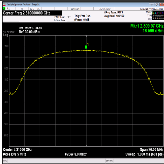
40(2305-2315)-10MHz-16QAM-38750-50RB#0-PASS
