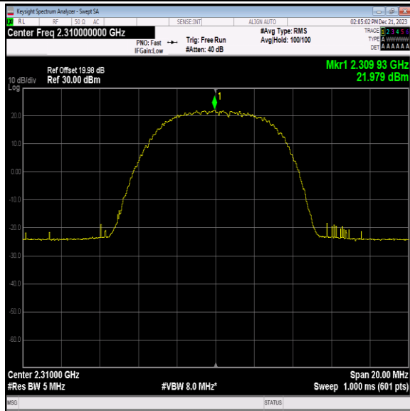
40(2305-2315)-10MHz-QPSK-38750-1RB#24-PASS
