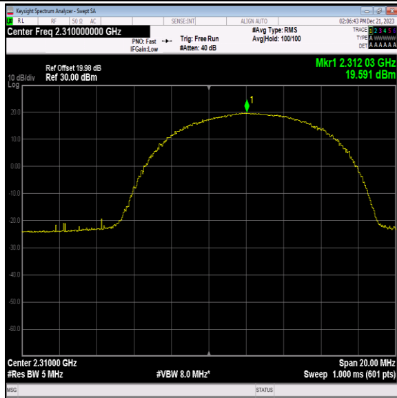
40(2305-2315)-10MHz-QPSK-38750-25RB#25-PASS
