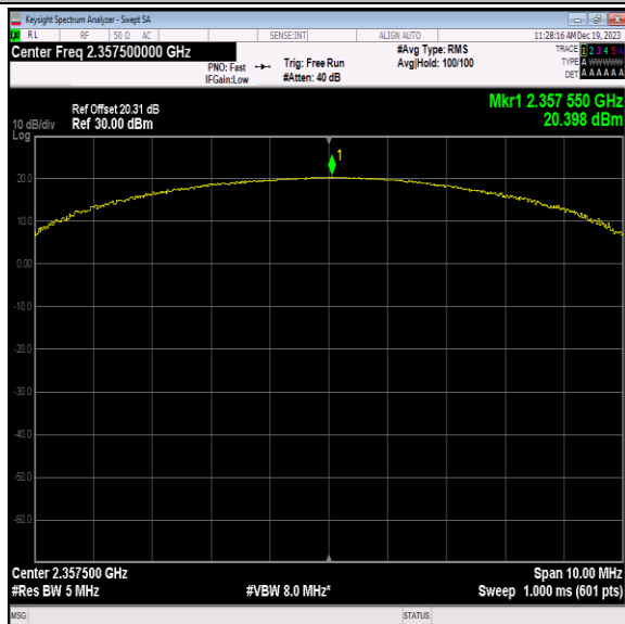
40(2350-2360)-5MHz-QPSK-39225-25RB#12-PASS
