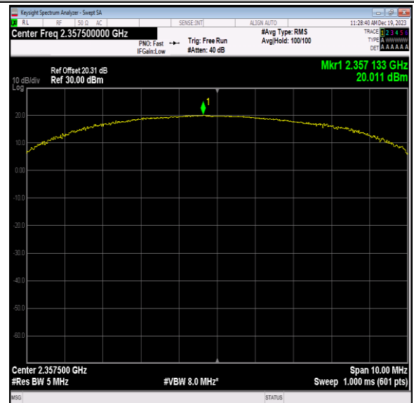
40(2350-2360)-5MHz-QPSK-39225-25RB#25-PASS
