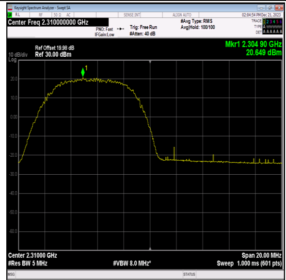
40(2305-2315)-10MHz-64QAM-38750-1RB#0-PASS
