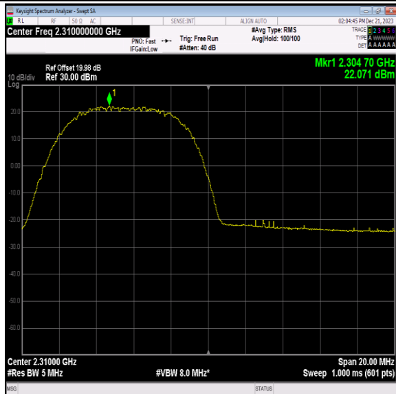
40(2305-2315)-10MHz-16QAM-38750-1RB#0-PASS
