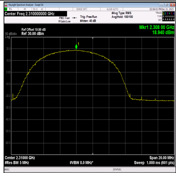
40(2305-2315)-10MHz-16QAM-38750-25RB#0-PASS
