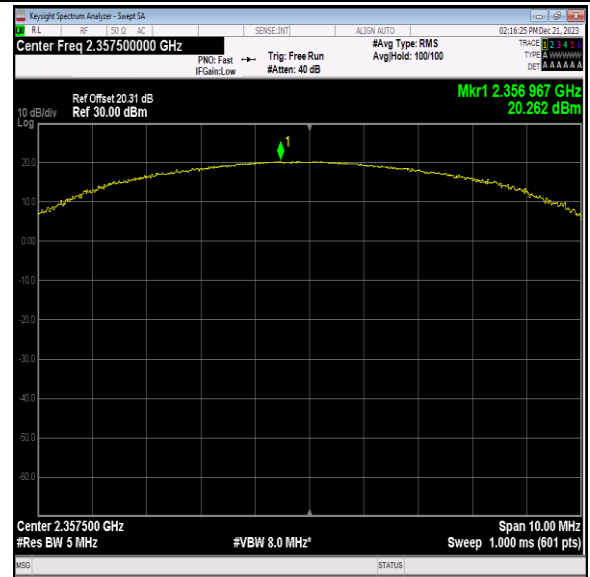
40(2350-2360)-5MHz-QPSK-39225-25RB#0-PASS
