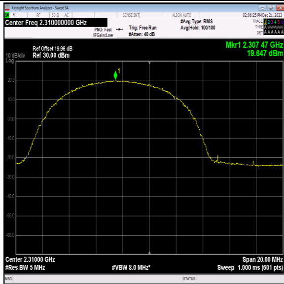
40(2305-2315)-10MHz-16QAM-38750-25RB#12-PASS
