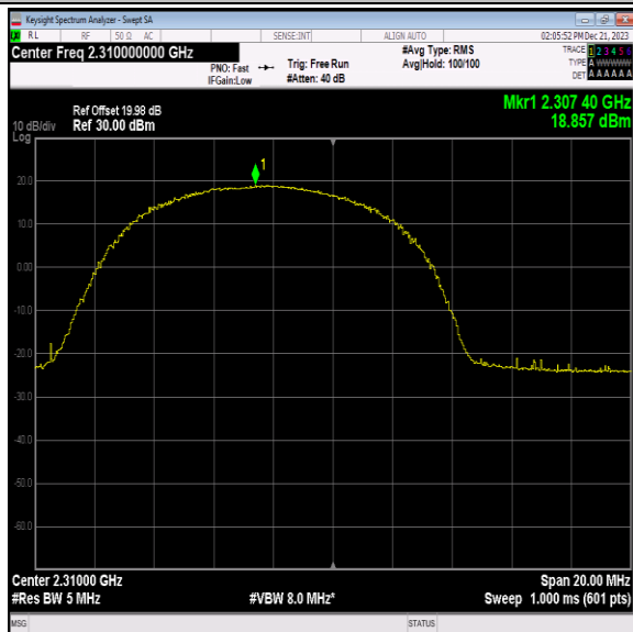
40(2305-2315)-10MHz-QPSK-38750-25RB#0-PASS
