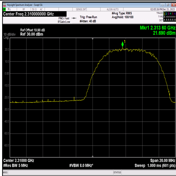
40(2305-2315)-10MHz-16QAM-38750-1RB#49-PASS
