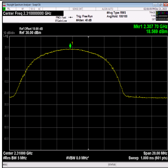
40(2305-2315)-10MHz-64QAM-38750-25RB#0-PASS
