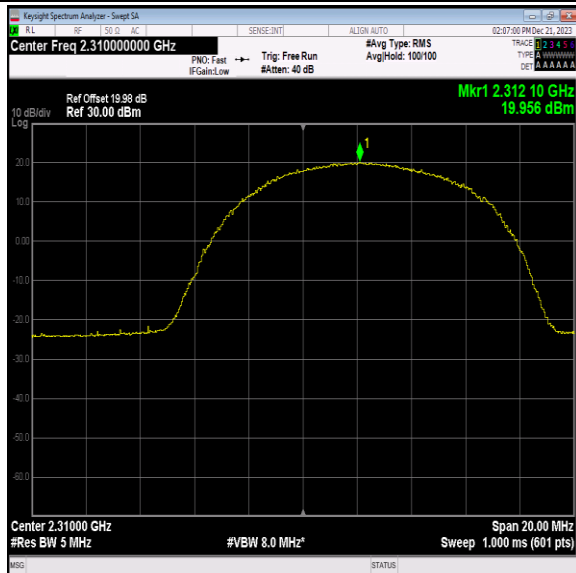
40(2305-2315)-10MHz-64QAM-38750-25RB#25-PASS
