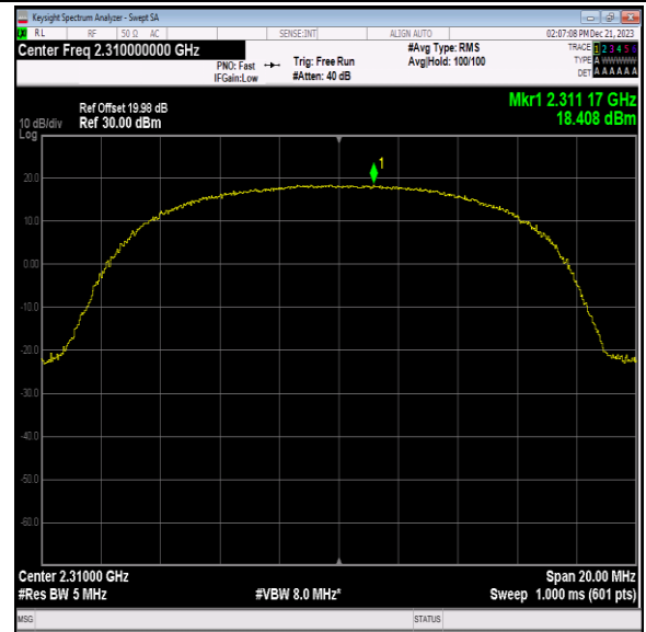
40(2305-2315)-10MHz-QPSK-38750-50RB#0-PASS
