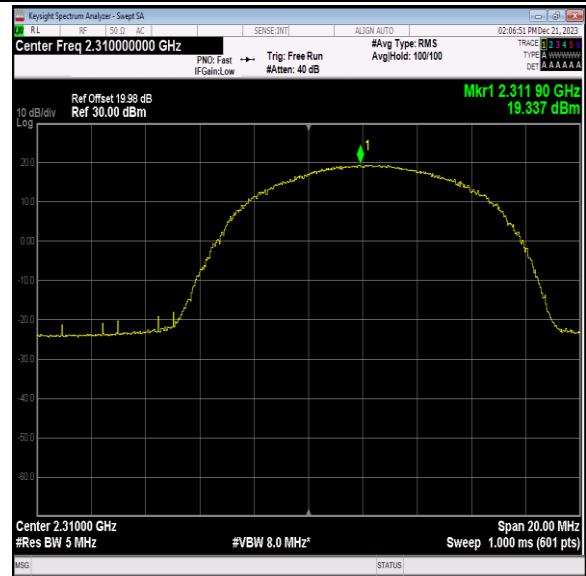
40(2305-2315)-10MHz-16QAM-38750-25RB#25-PASS
