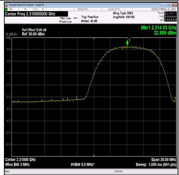
40(2305-2315)-10MHz-QPSK-38750-1RB#49-PASS
