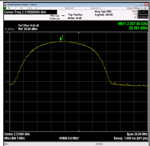
40(2305-2315)-10MHz-QPSK-38750-25RB#12-PASS
