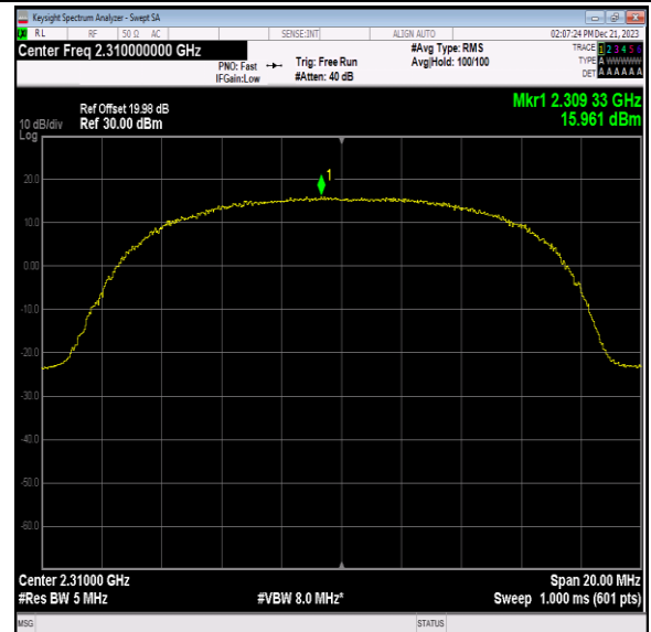
40(2305-2315)-10MHz-64QAM-38750-50RB#0-PASS
