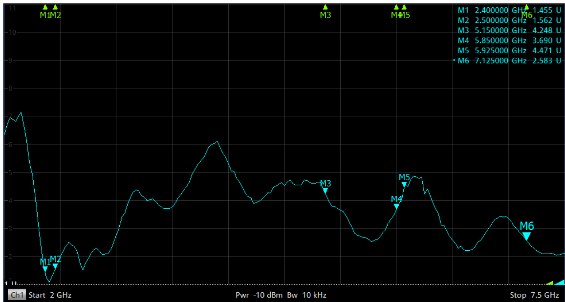
WiFi1 2.4GHz Antenna
