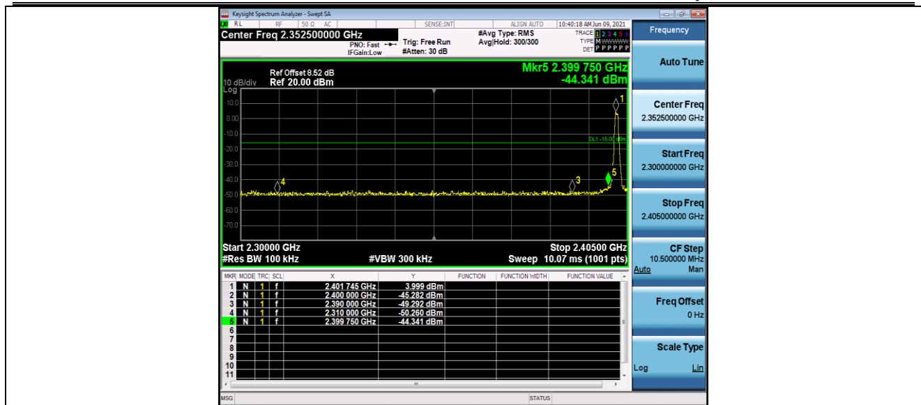
BLE_500K_Ant1_Low_2402
