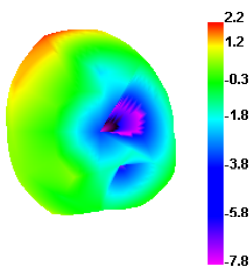
2450.000MHz
