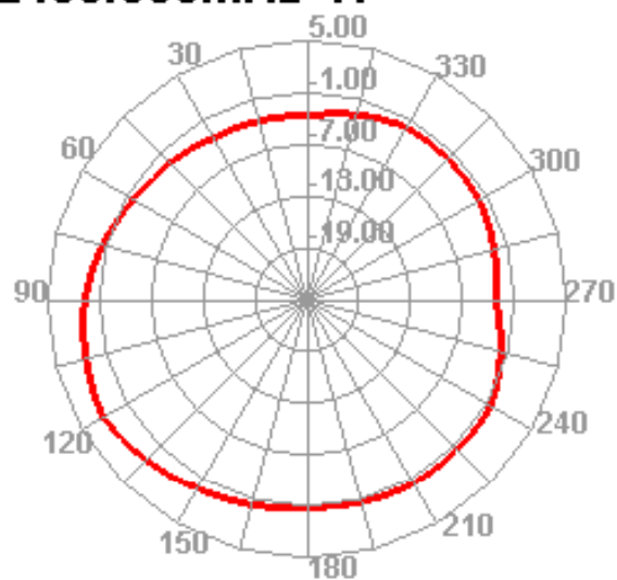
2450.000MHz H
