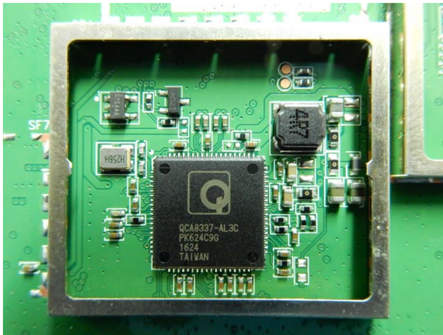
(19) EUT Photo
