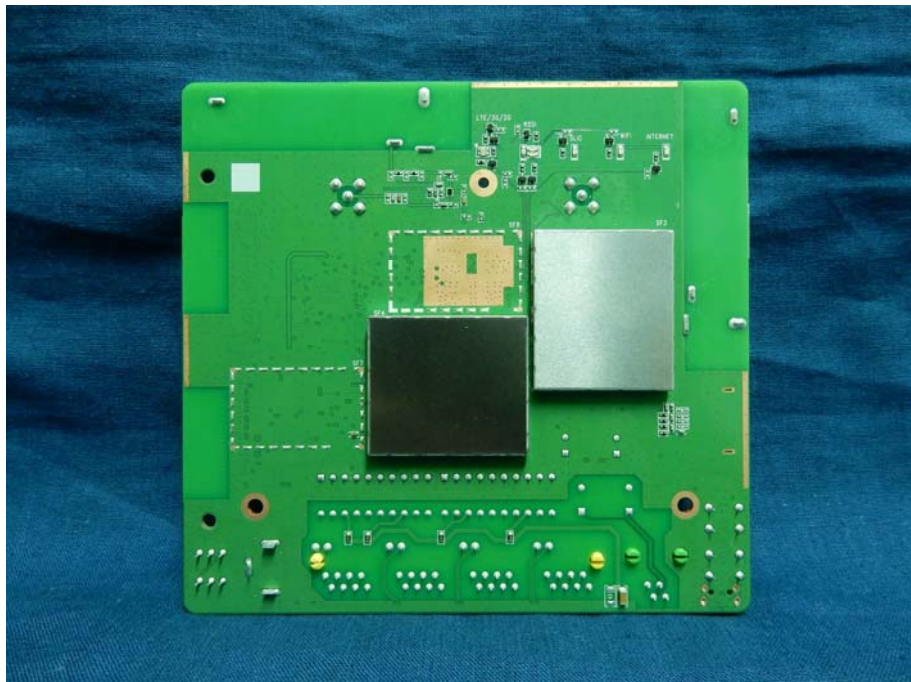
(16) EUT Photo
