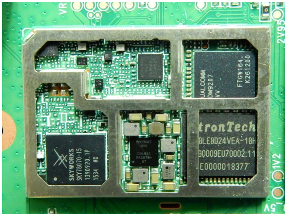
(15) EUT Photo
