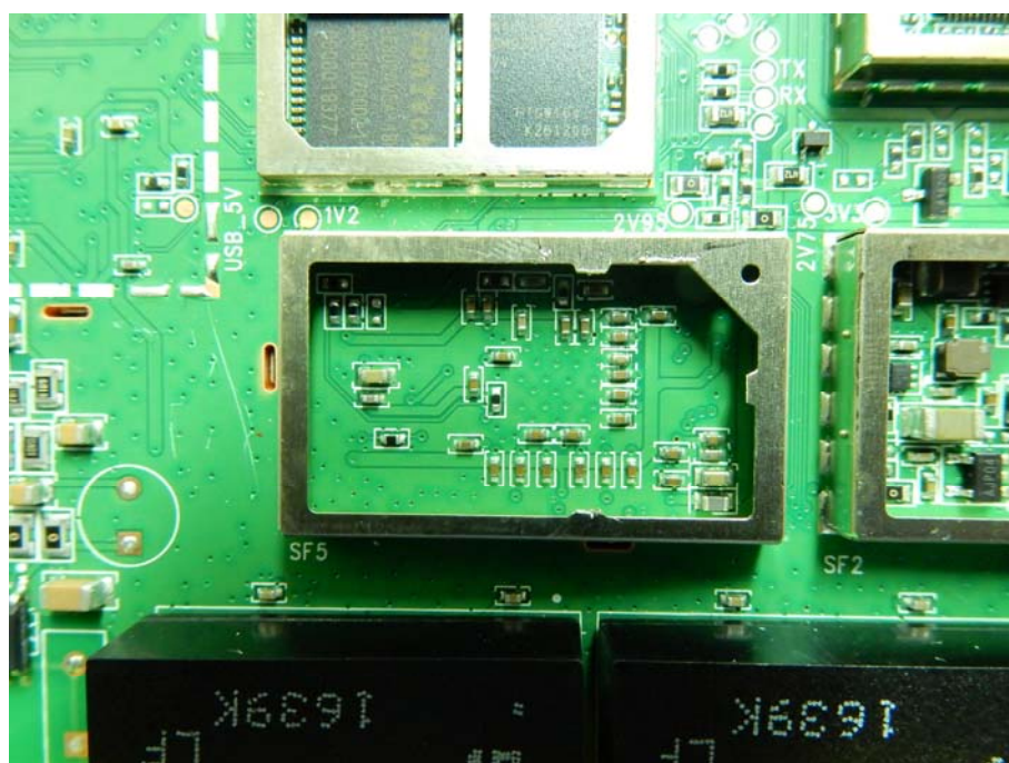
(14) EUT Photo
