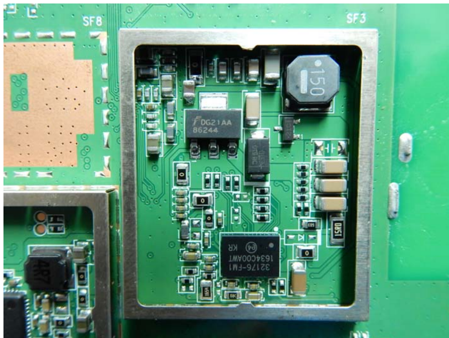
(20) EUT Photo
