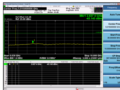
B13-5M-Low CH-CSE-1-Q16-1 RB 0
