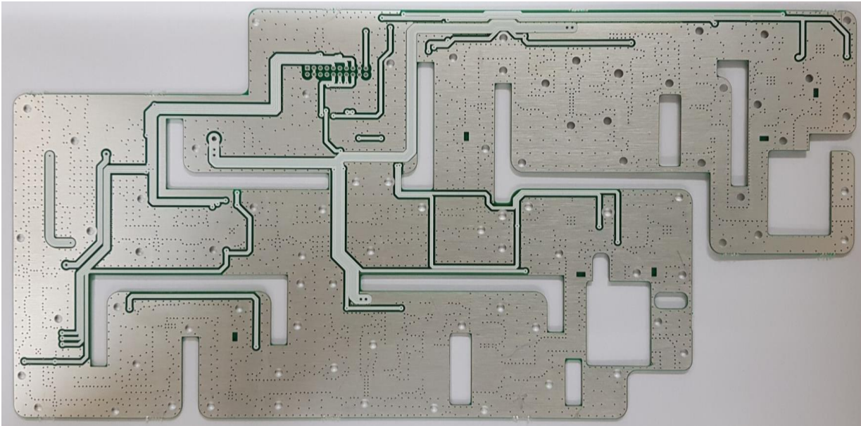
TX PCB Bottom
