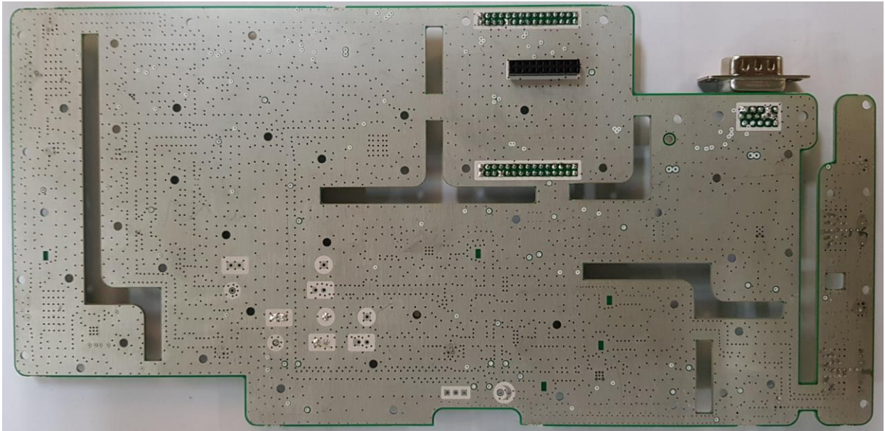
RX PBA Bottom
