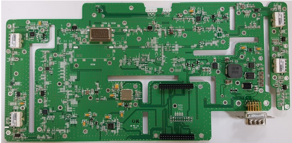
RX PBA Top
