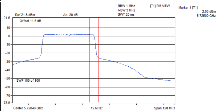
802.11be (EHT40) / Chain 2 : CH 142 (U-NII-3)
