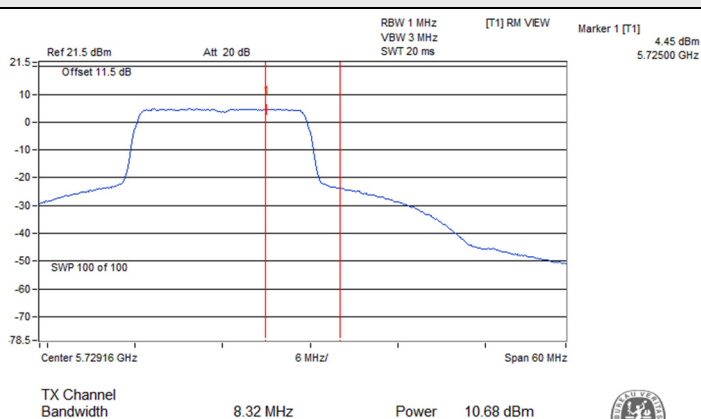
802.11be (EHT20) / Chain 2 : CH 144 (U-NII-3)
