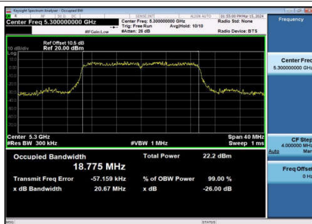
U-NII-2a 99%&amp;26dB Bandwidth-802.11ax(20MHz),5300MHz,Ant1
