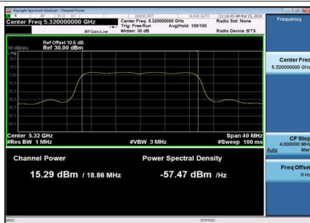
U-NII-2a Output Power-802.11ax(20MHz) ,5320MHz,Ant1
