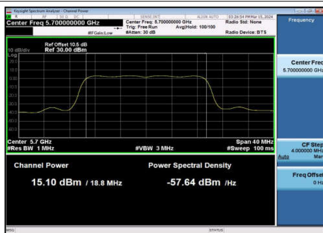
U-NII-2c Output Power-802.11ax(20MHz) ,5700MHz,Ant1
