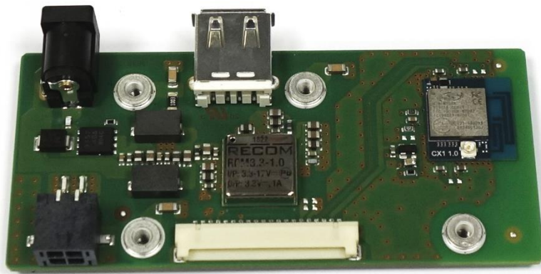
Top view PCBA Redpine WLAN Module
