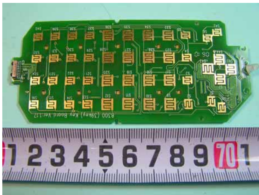
24keys keypad
