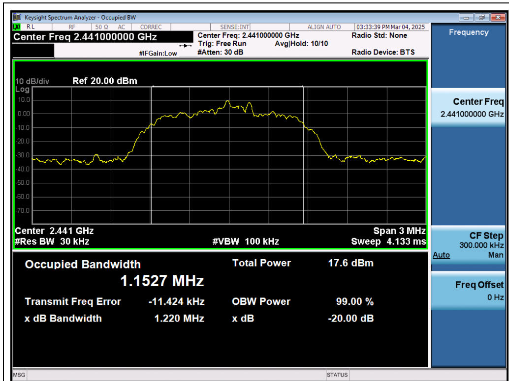
Test_Graph_EDR_ANT1_2441_2Mbps_OBW
