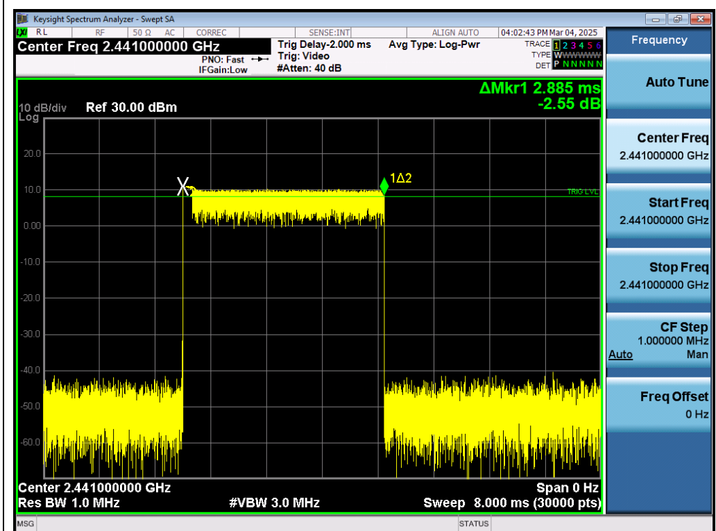
Test_Graph_EDR_HOP_ANT1_NA_2Mbps_2441_Time per Burst
