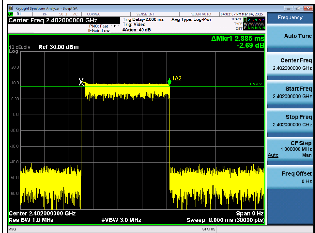
Test_Graph_EDR_HOP_ANT1_NA_2Mbps_2402_Time per Burst
