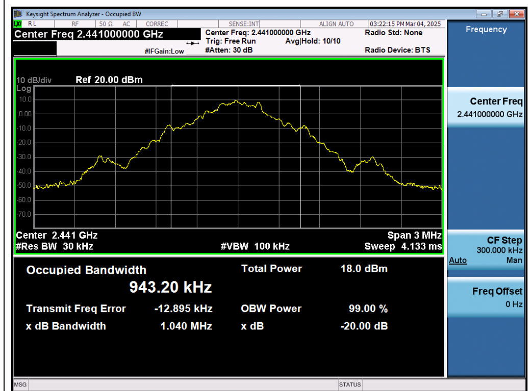
Test_Graph_BR_ANT1_2441_1Mbps_OBW
