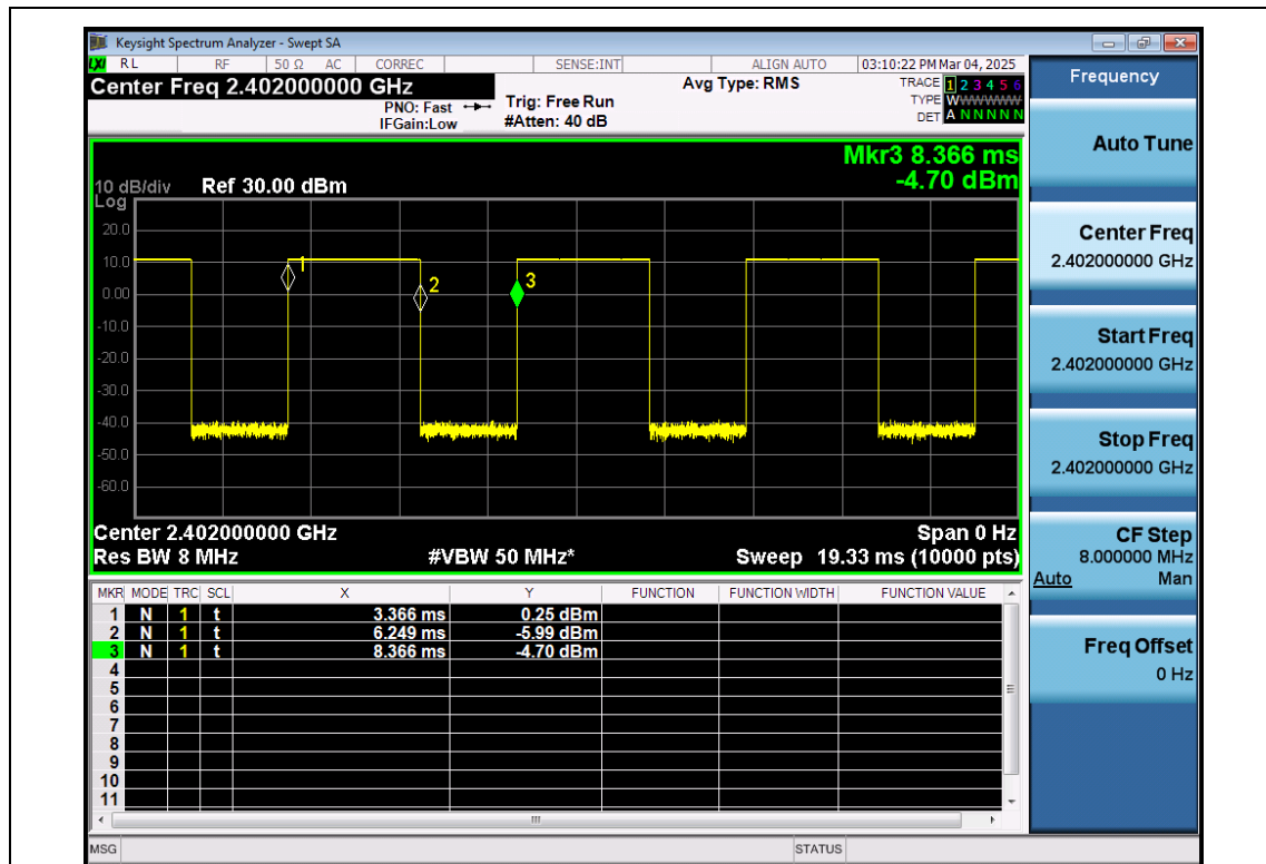
BR-GFSK-ANT1-2402
