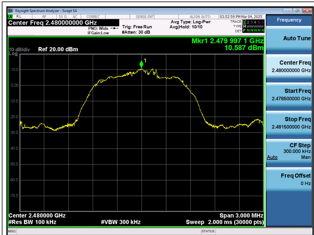
Test_Graph_EDR_ANT1_2480_3Mbps_Reference Level
