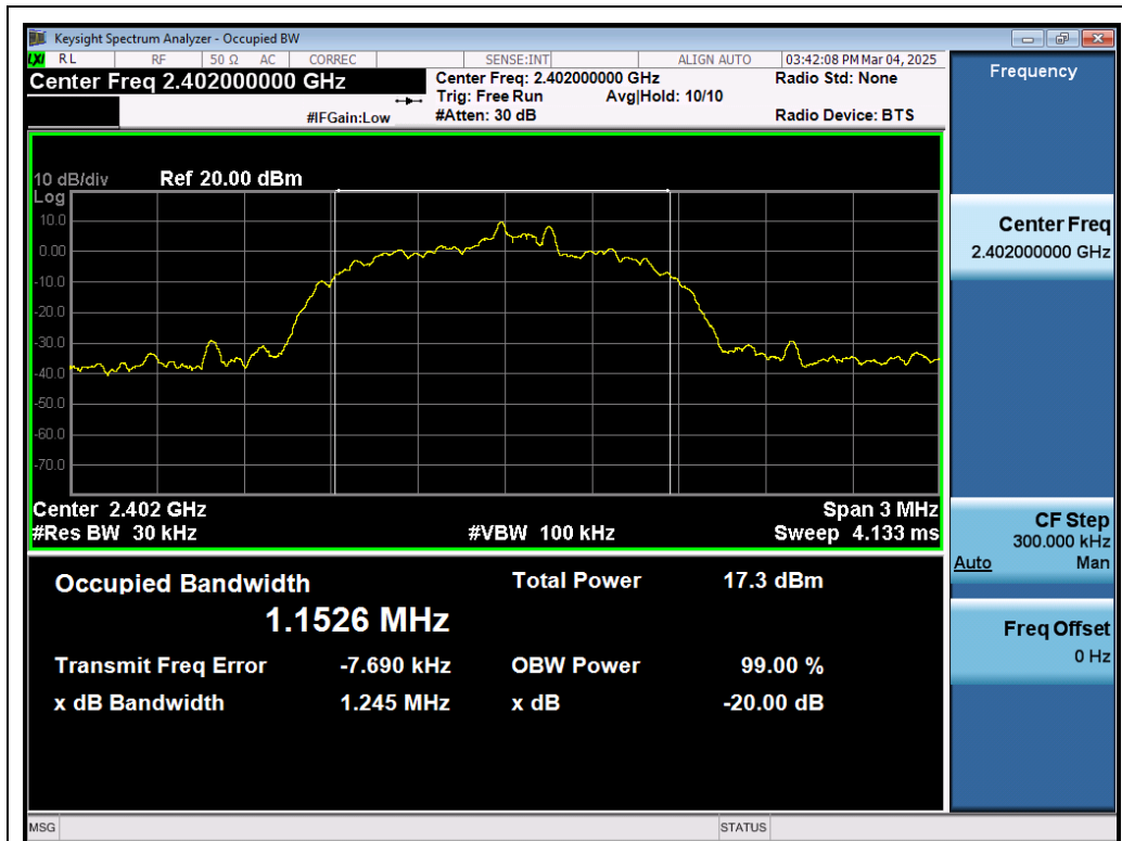
Test_Graph_EDR_ANT1_2402_3Mbps_OBW
