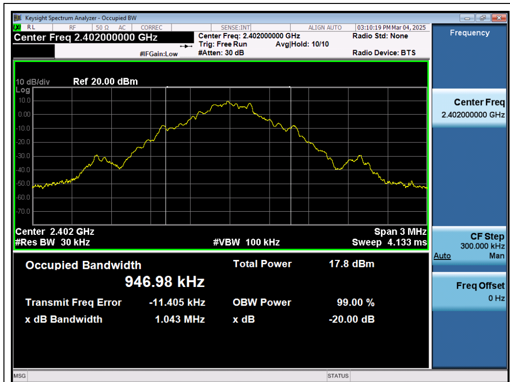
Test_Graph_BR_ANT1_2402_1Mbps_OBW
