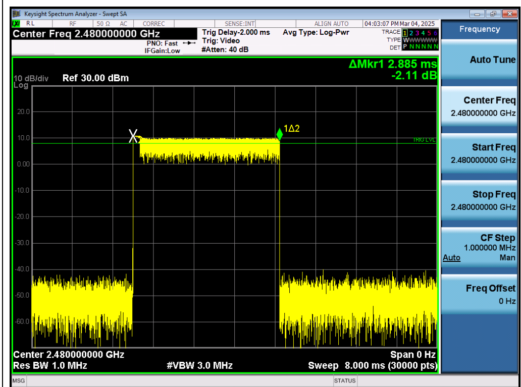
Test_Graph_EDR_HOP_ANT1_NA_2Mbps_2480_Time per Burst
