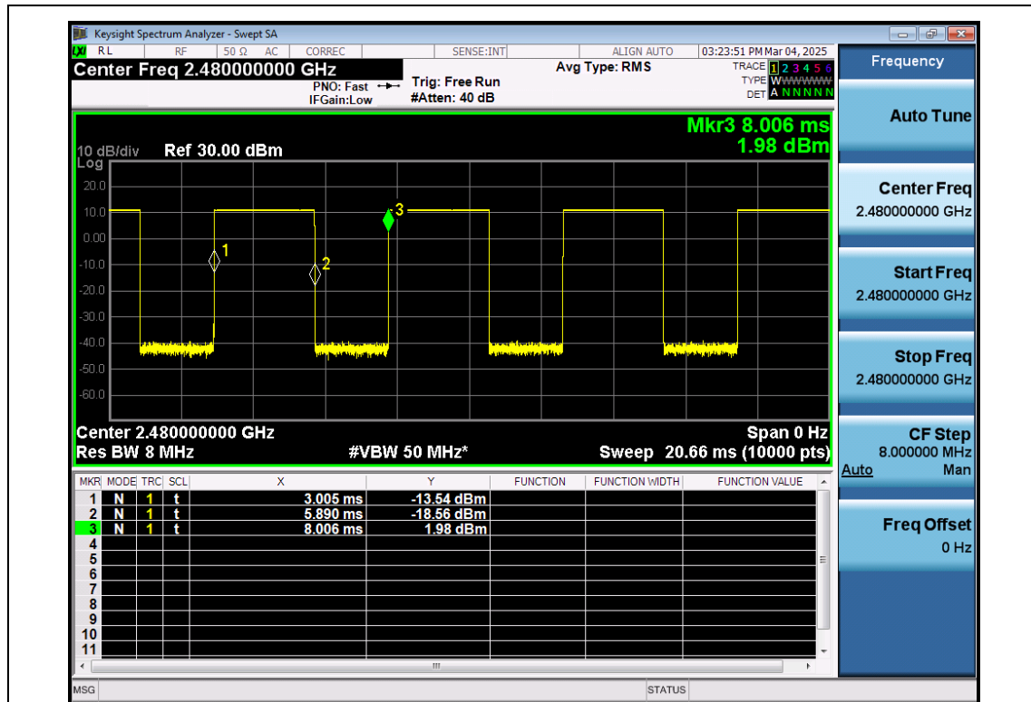
BR-GFSK-ANT1-2480
