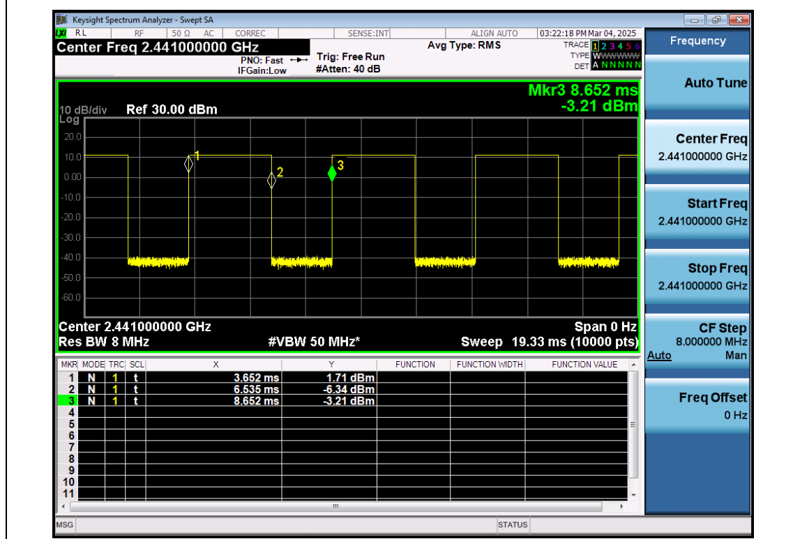
BR-GFSK-ANT1-2441
