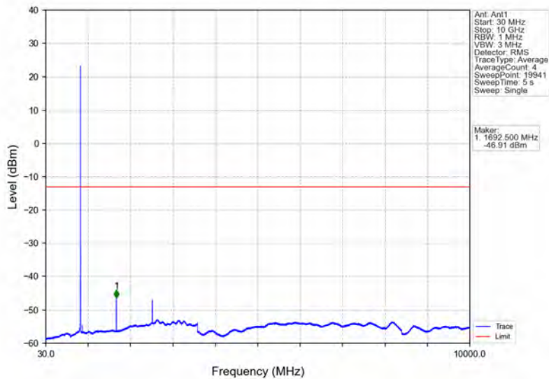
Band26b_3MHz_QPSK_HCH_847.5MHz_RB_1_14_NTNV
