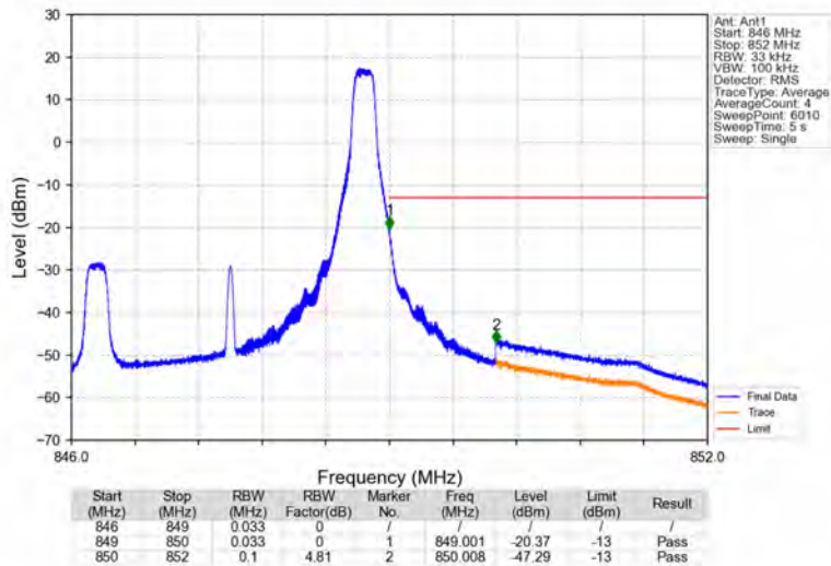
Band26b_3MHz_QPSK_HCH_847.5MHz_RB_1_14_NTNV
