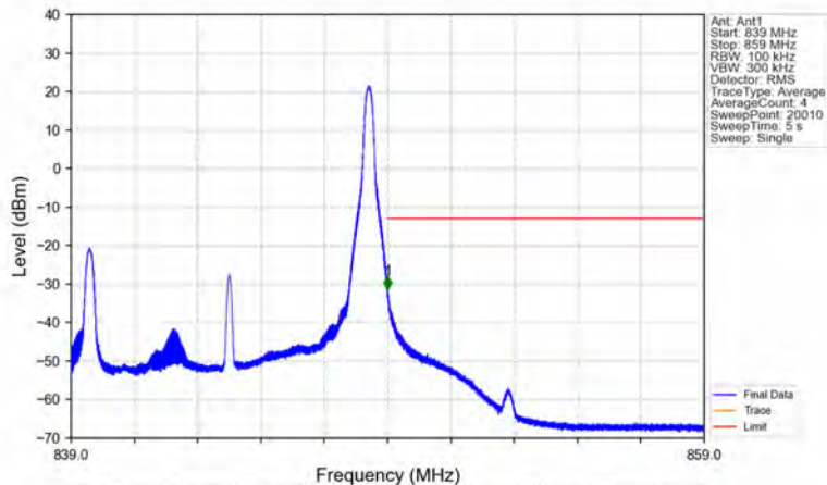
Band26b_10MHz_QPSK_HCH_844MHz_RB_1_49_NTNV
