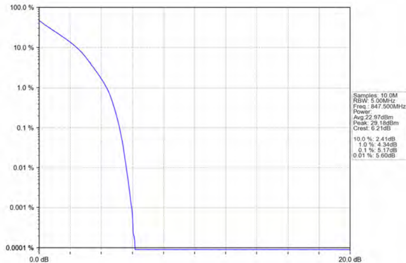
Band26b_3MHz_QPSK_HCH_847.5MHz_RB_15_0_NTNV
