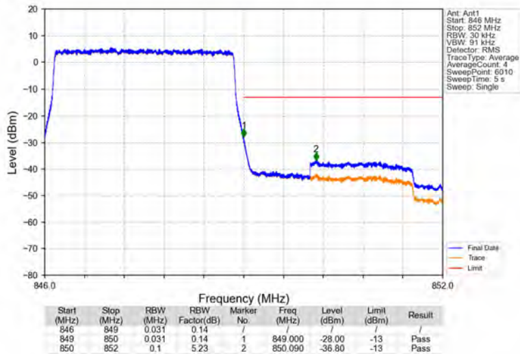
Band26b_3MHz_QPSK_HCH_847.5MHz_RB_15_0_NTNV
