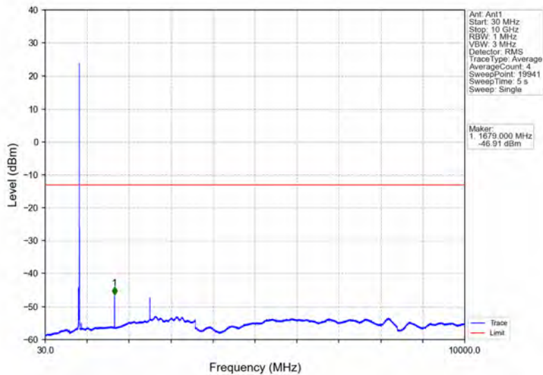
Band26b_10MHz_QPSK_HCH_844MHz_RB_1_49_NTNV
