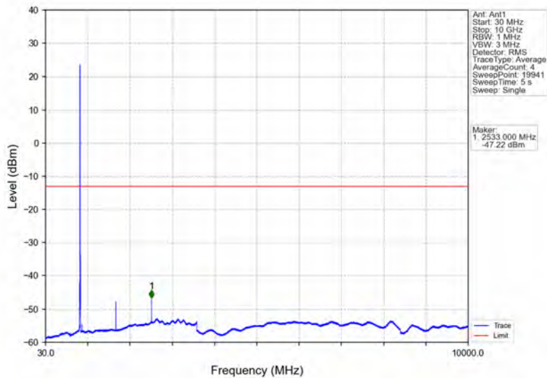
Band26b_5MHz_QPSK_HCH_846.5MHz_RB_1_24_NTNV
