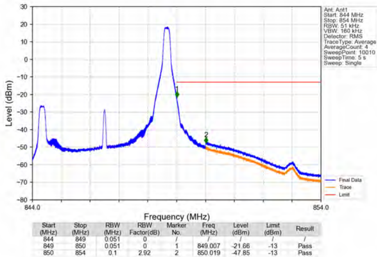
Band26b_5MHz_QPSK_HCH_846.5MHz_RB_1_24_NTNV
