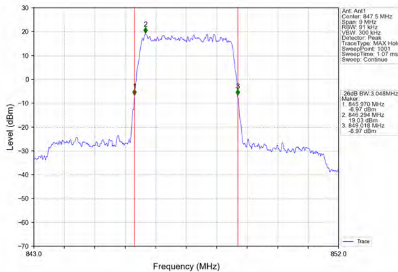
Band26b_3MHz_QPSK_HCH_847.5MHz_RB_15_0_NTNV
