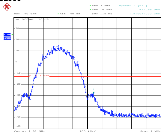
EGPRS1900
