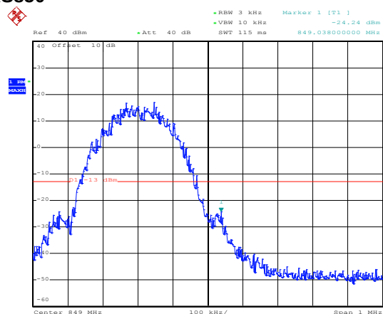
EGPRS850
