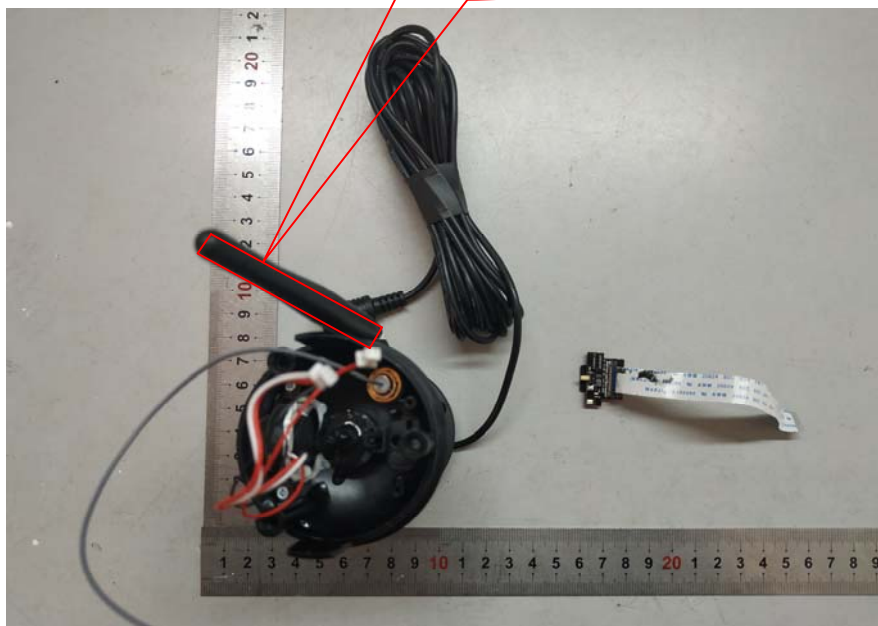
Omni Antenna
