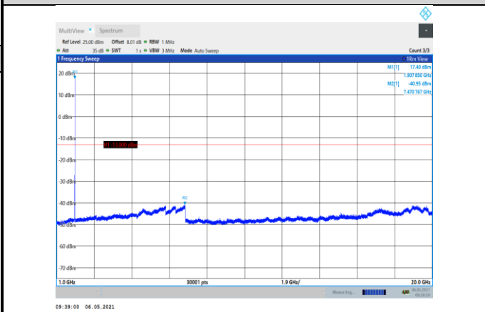
Band2-9538-1000~20000MHz
