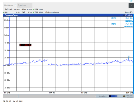
Band2-1.4MHz-QPSK-19193-1RB#0- Range2:1000~20000MHz
