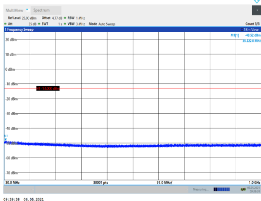
Band4-1413-30~1000MHz
