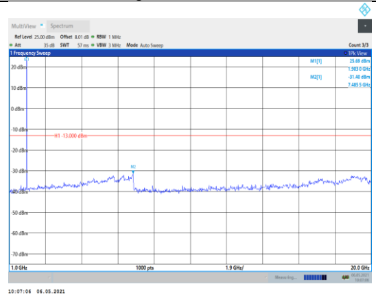
Band2-3MHz-QPSK-19185-1RB#0- Range2:1000~20000MHz
