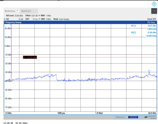
Band2-10MHz-QPSK-19150-1RB#0- Range2:1000~20000MHz
