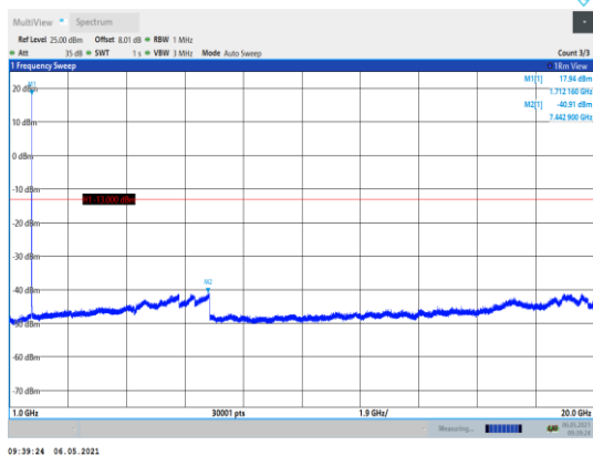
Band4-1312-1000~20000MHz
