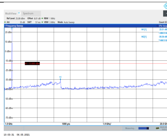
Band2-5MHz-QPSK-18900-1RB#0- Range2:1000~20000MHz
