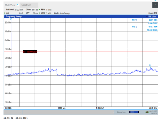
Band2-1.4MHz-QPSK-18900-1RB#0- Range2:1000~20000MHz
