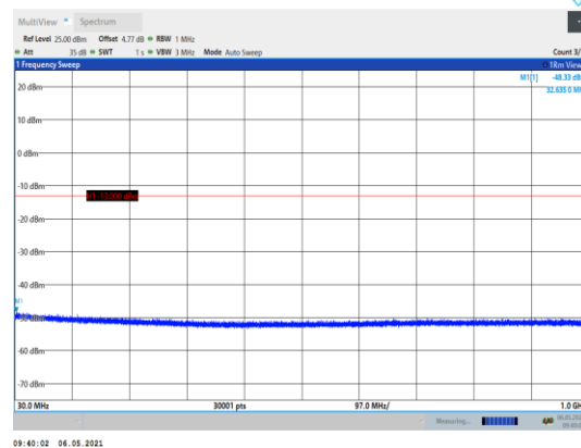
Band4-1513-30~1000MHz
