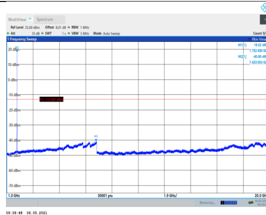
Band4-1413-1000~20000MHz
