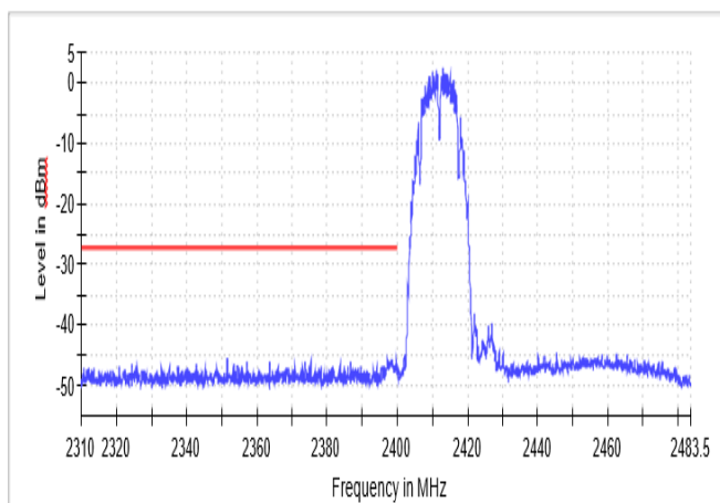
Band Edge
