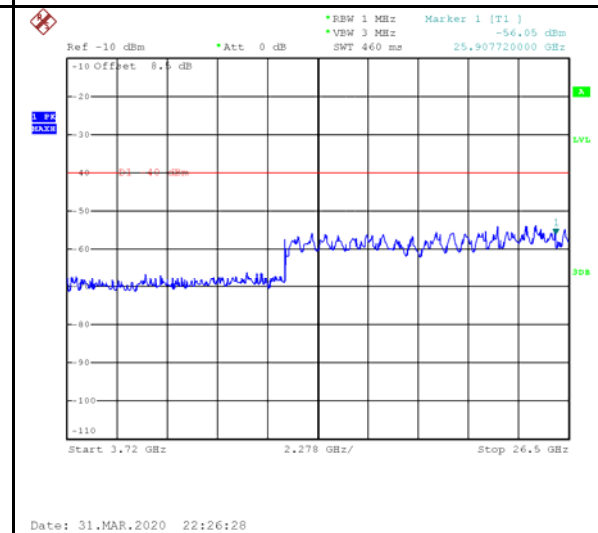
5MHz - High CH 3.72GHz~26.5GHz
