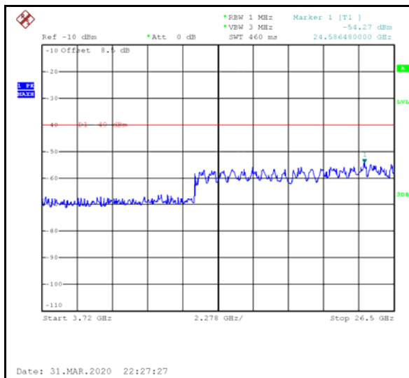
20MHz - Low CH 3.72GHz~26.5GHz
