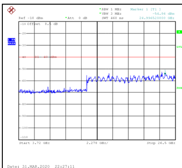
15MHz - Middle CH 3.72GHz~26.5GHz
