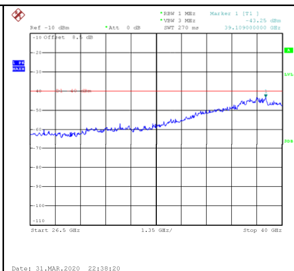
10MHz - Low CH 26.5GHz~40GHz
