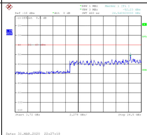
15MHz - High CH 3.72GHz~26.5GHz
