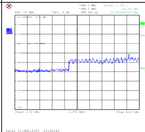
10MHz - Middle CH 3.72GHz~26.5GHz
