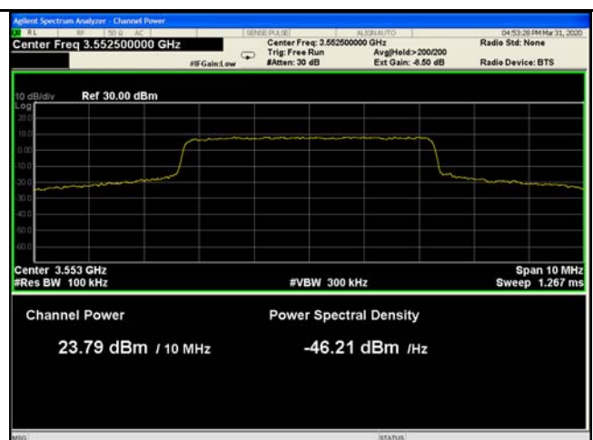
5MHz - Low CH 16QAM
