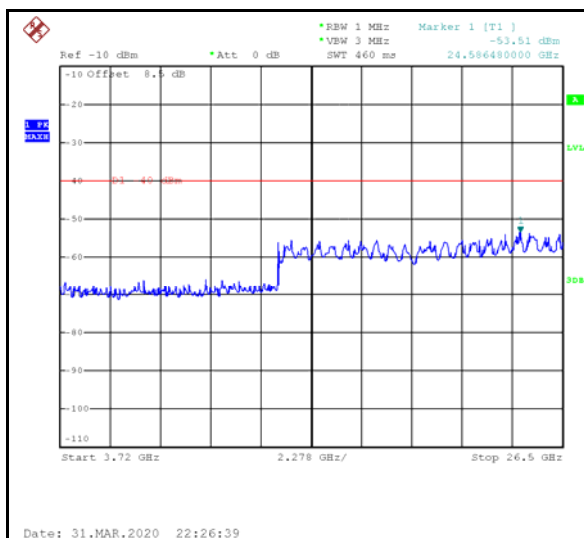
10MHz - Low CH 3.72GHz~26.5GHz
